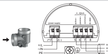
Aansluitruimte tweekamerbehuizing - netspanning
