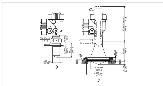
Afmetingen VEGAPULS 61
