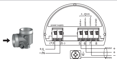
Aansluitruimte tweekamerbehuizing - laagspanning
