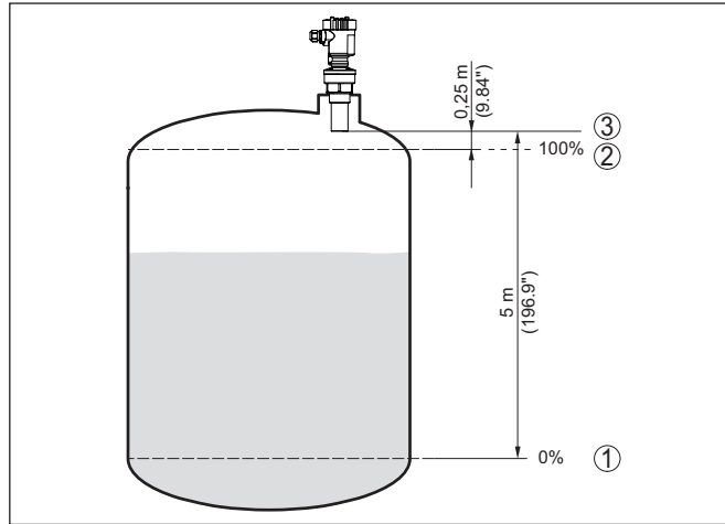
Abb. 7: Parametrierbeispiel Min.-/Max.-Abgleich
