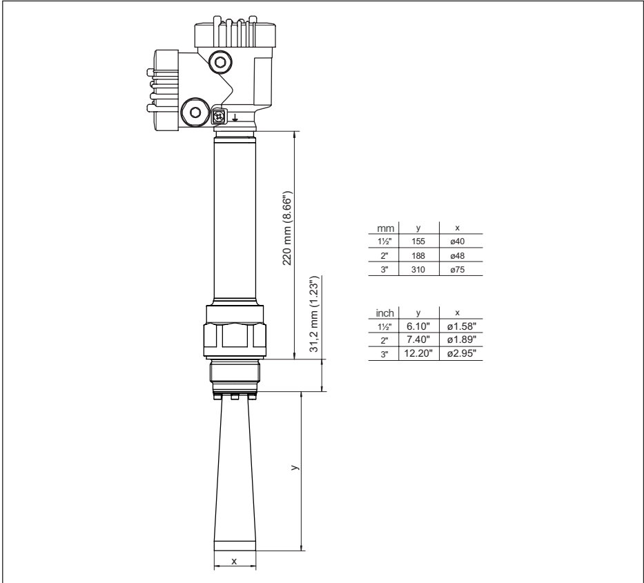
Abb. 89: VEGAPULS 6X, Gewinde mit Hornantenne 450 °C-Ausführung
