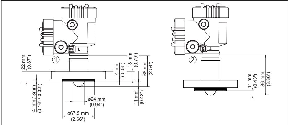
Abb. 91: VEGAPULS 6X, gekapseltes Antennensystem DN 25 PN 40
