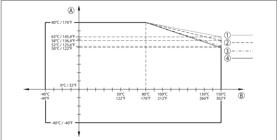
Abb. 72: Derating Umgebungstemperatur, Flansch mit Linsenantenne bis +150 °C (+302 °F)
