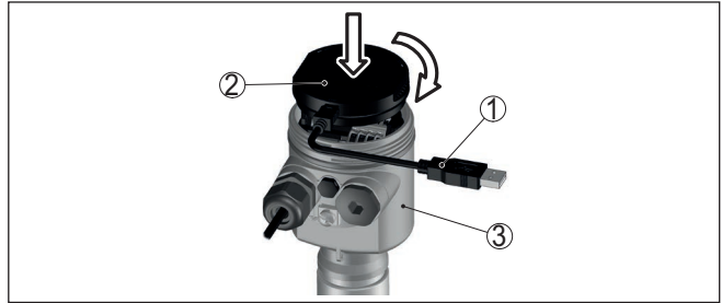
Abb. 57: Anschluss des PCs via Schnittstellenadapter direkt am Sensor
