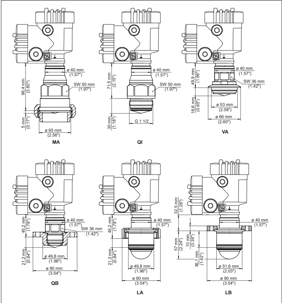
Abb. 95: VEGAPULS 6X, Hygieneanschluss
