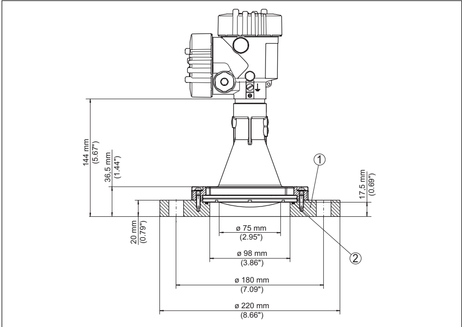
Abb. 82: VEGAPULS 6X mit Adapterflansch DN 100 PN 6
