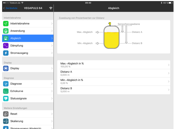
Abb. 54: Beispielf einer App-Ansicht - Inbetriebnahme Messwerte
