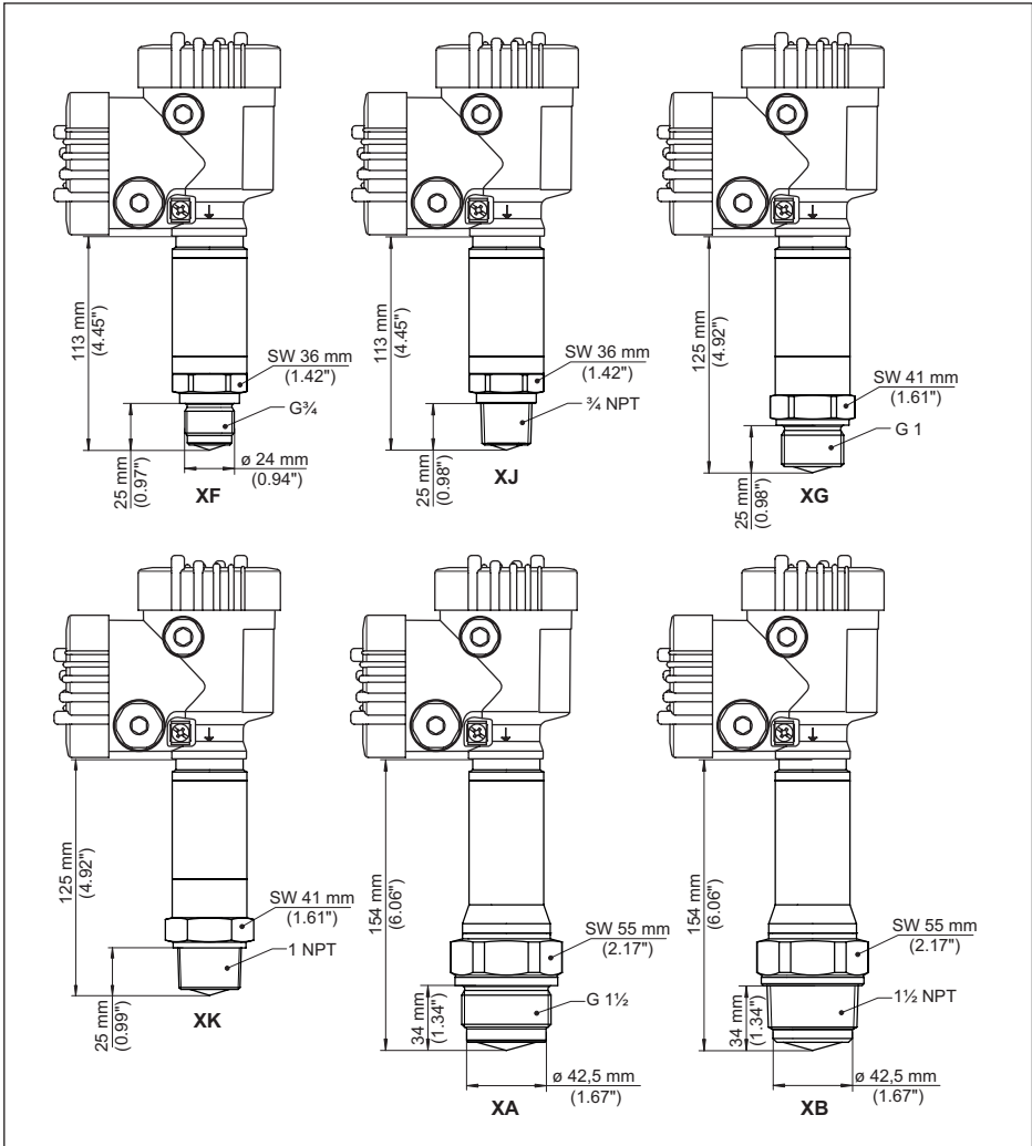
Abb. 87: VEGAPULS 6X, Gewinde mit integriertem Antennensystem bis +200 °C (+392 °F) und +250 °C (+482 °F)
