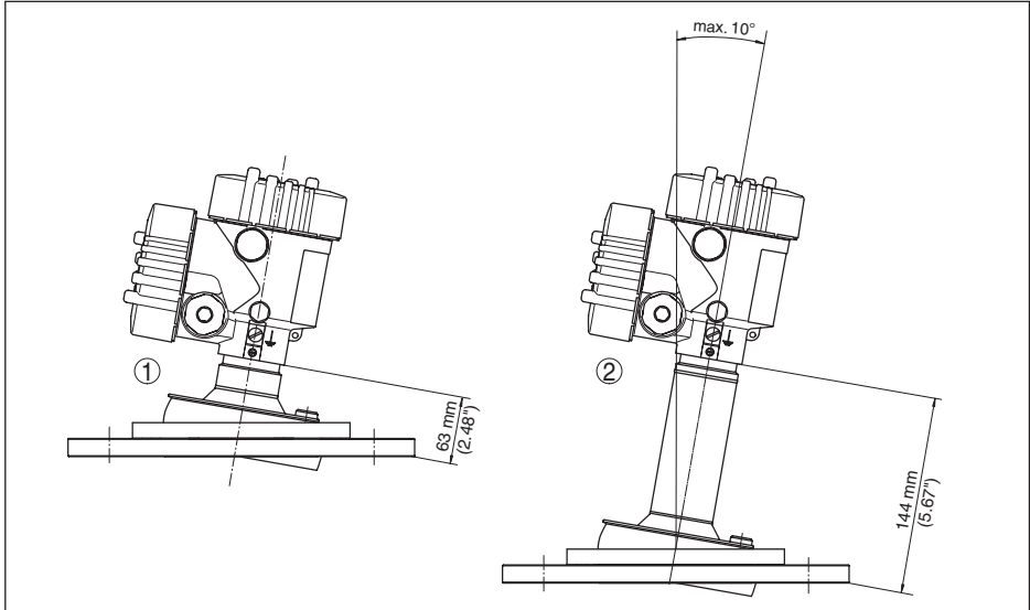
Abb. 98: VEGAPULS 6X, Flansch mit Linsenantenne und Schwenkhalterung
