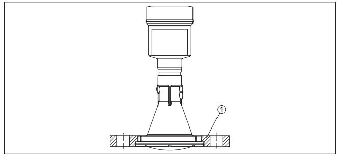
Abb. 13: Kombi-Überwurfflansch
