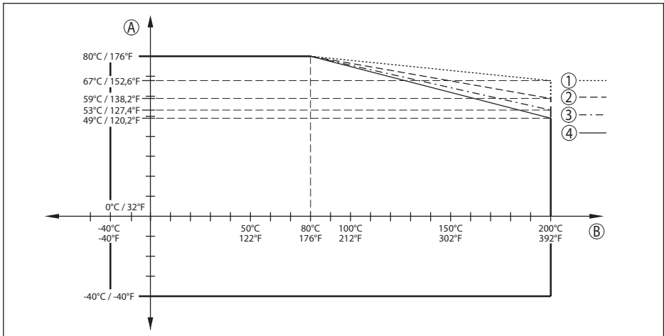
Abb. 77: Derating Umgebungstemperatur, Flansch mit Hornantenne bis +200 °C (+392 °F)
