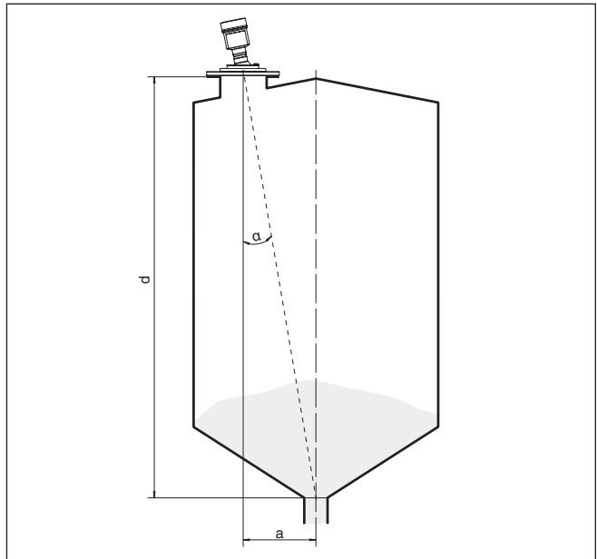
Abb. 32: Ermittlung des Neigungswinkels zur Ausrichtung des VEGAPULS 6X
