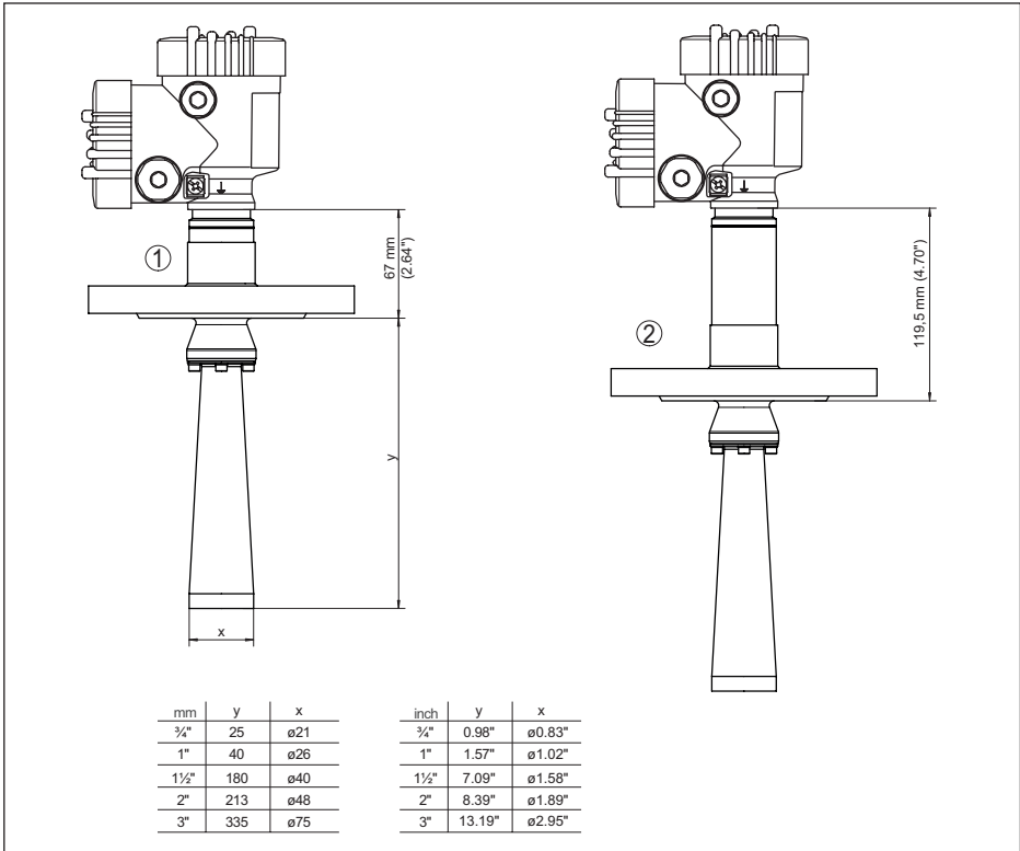
Abb. 88: VEGAPULS 6X, Flansch mit Hornantenne bis +150 °C (+302 °F)/+250 °C (+482 °F)
