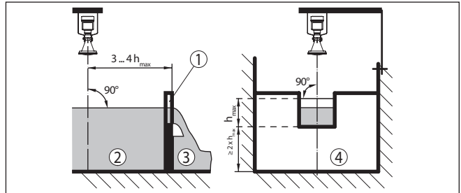
Abb. 42: Durchflussmessung mit Rechtecküberfall: h_{\text{max}} = \text{max. Befüllung des Rechtecküberfalls}
