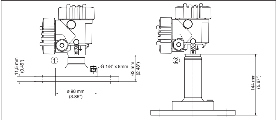
Abb. 96: VEGAPULS 6X, Flansch mit Linsenantenne (Flanschstärke siehe Zeichnung, Flanschmaße nach DIN, ASME, JIS)
