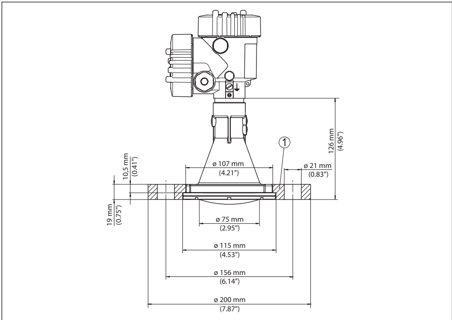
Abb. 80: VEGAPULS 6X mit Überwurfflansch passend für 3" 150 lbs, DN 80 PN 16
