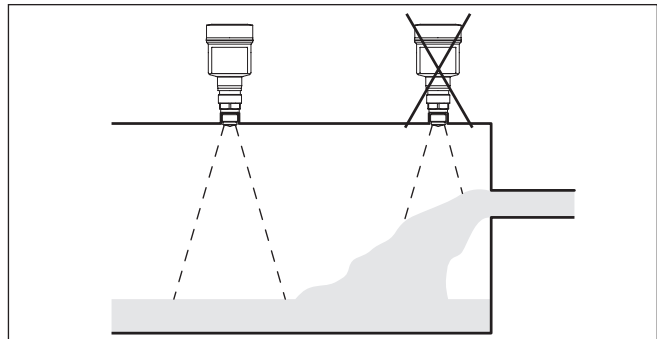
Abb. 20: Montage des Radarsensors bei einströmendem Medium
