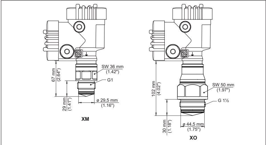
Abb. 93: VEGAPULS 6X, Gewinde für Hygieneadapter
