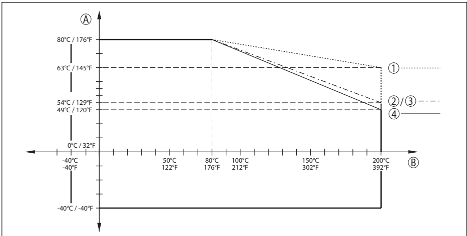
Abb. 73: Derating Umgebungstemperatur, Flansch mit Linsenantenne bis +200 °C (+392 °F)
