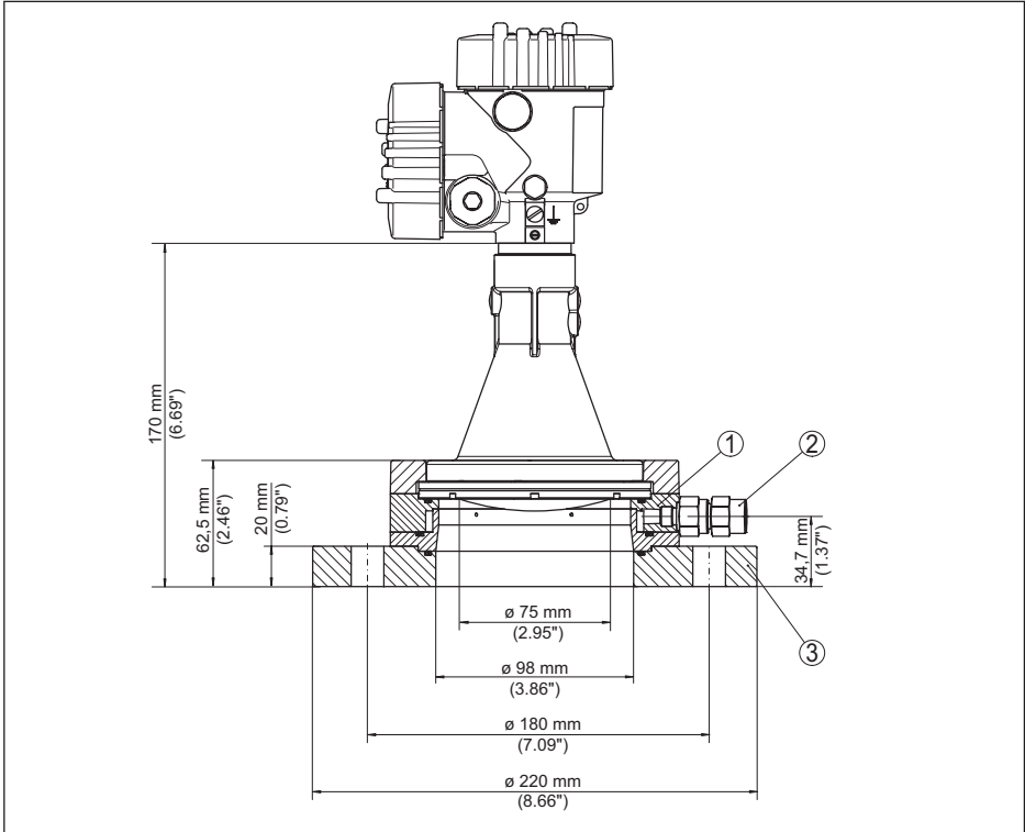
Abb. 83: VEGAPULS 6X, Adapterflansch und Spülluftanschluss DN 100 PN 6
