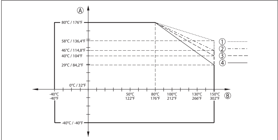
Abb. 76: Derating Umgebungstemperatur, Flansch mit Hornantenne bis +150 °C (+302 °F)
