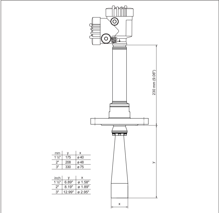
Abb. 90: VEGAPULS 6X, Flansch mit Hornantenne 450 °C-Ausführung
