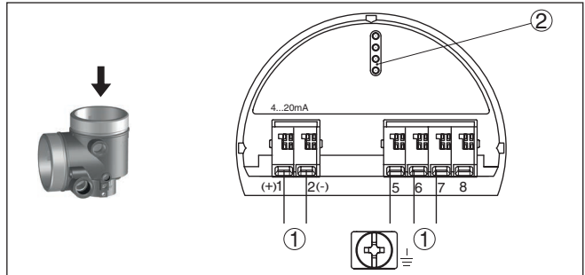
Abb. 45: Elektronikraum - Zweikammergehäuse
