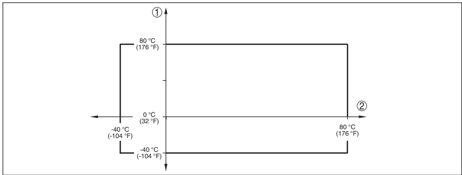
Abb. 64: Derating Umgebungstemperatur, Kunststoff-Hornantenne
