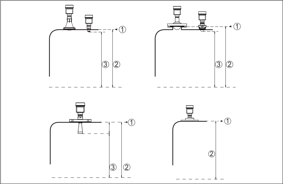
Abb. 62: Daten zur Eingangsgröße
