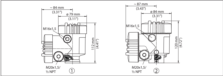
Abb. 79: VEGAPULS 6X; mit eingebautem Anzeige- und Bedienmodul vergrößert sich die Gehäusehöhe um 9 mm (0.35 in)
