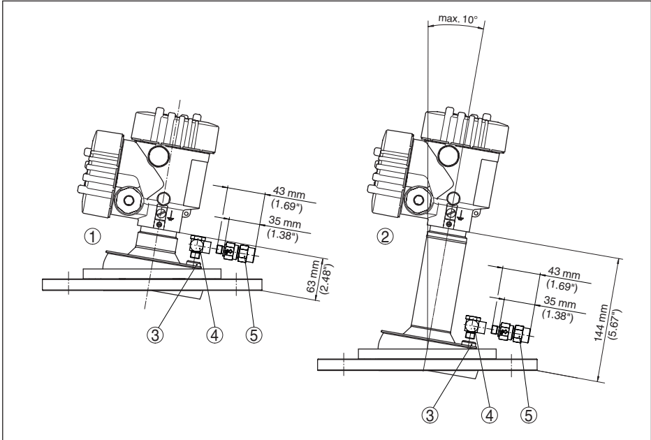
Abb. 99: VEGAPULS 6X, Flansch mit Linsenantenne, Schwenkhalterung und Spülluftanschluss
