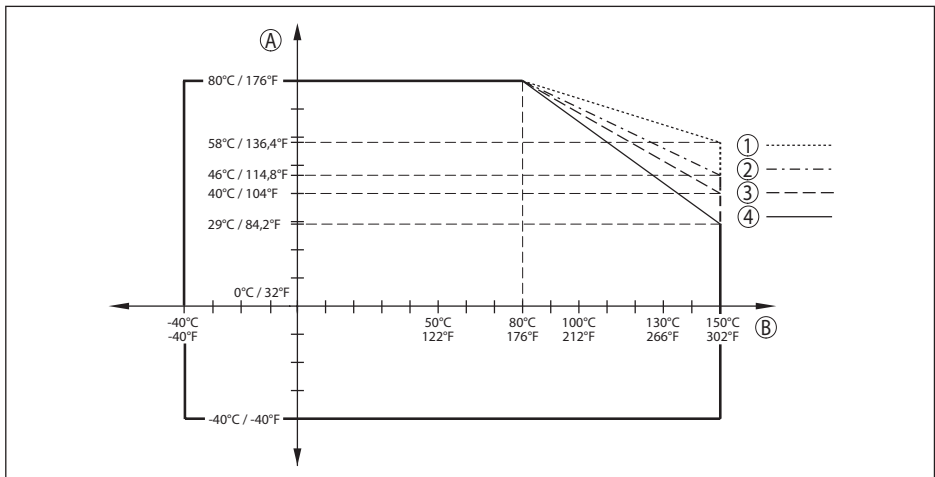
Abb. 65: Derating Umgebungstemperatur, Gewinde mit integriertem Antennensystem bis +150 °C (+302 °F)
