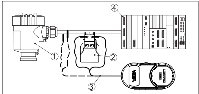
Abb. 58: Anschluss des PCs via HART an die Signalleitung
