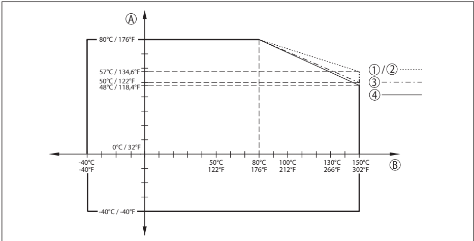
Abb. 68: Derating Umgebungstemperatur, Flansch mit gekapseltem Antennensystem bis +150 °C (+302 °F)
