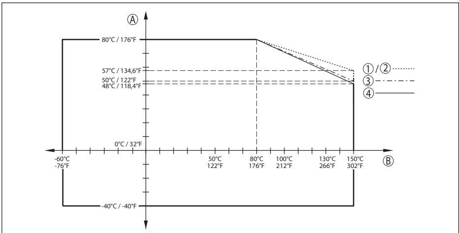
Abb. 69: Derating Umgebungstemperatur, Flansch mit gekapseltem Antennensystem -60 ... +150 °C (-76 ... +302 °F)
