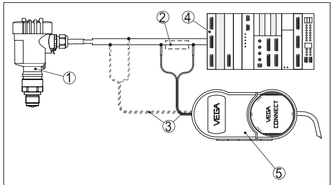
Abb. 3: Anschluss des PCs an die Signalleitung
