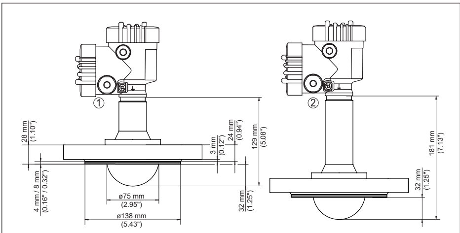
Abb. 92: VEGAPULS 6X, gekapseltes Antennensystem DN 80 PN 40
