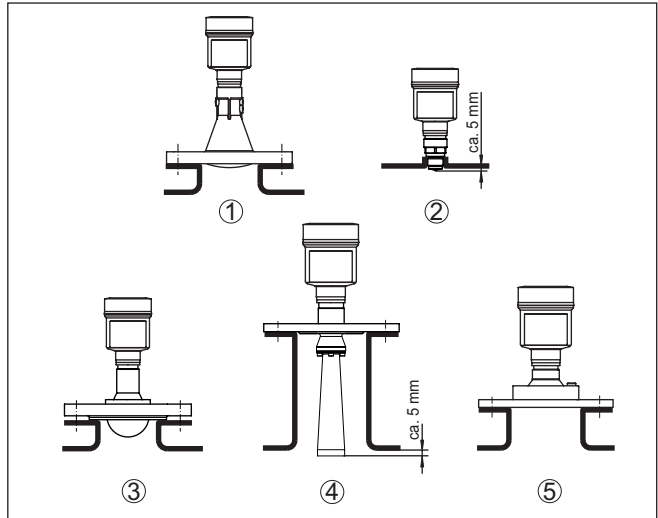
Abb. 23: Empfehlenswerte Rohrstützenmontage bei unterschiedlichen Ausführungen des VEGAPULS 6X
