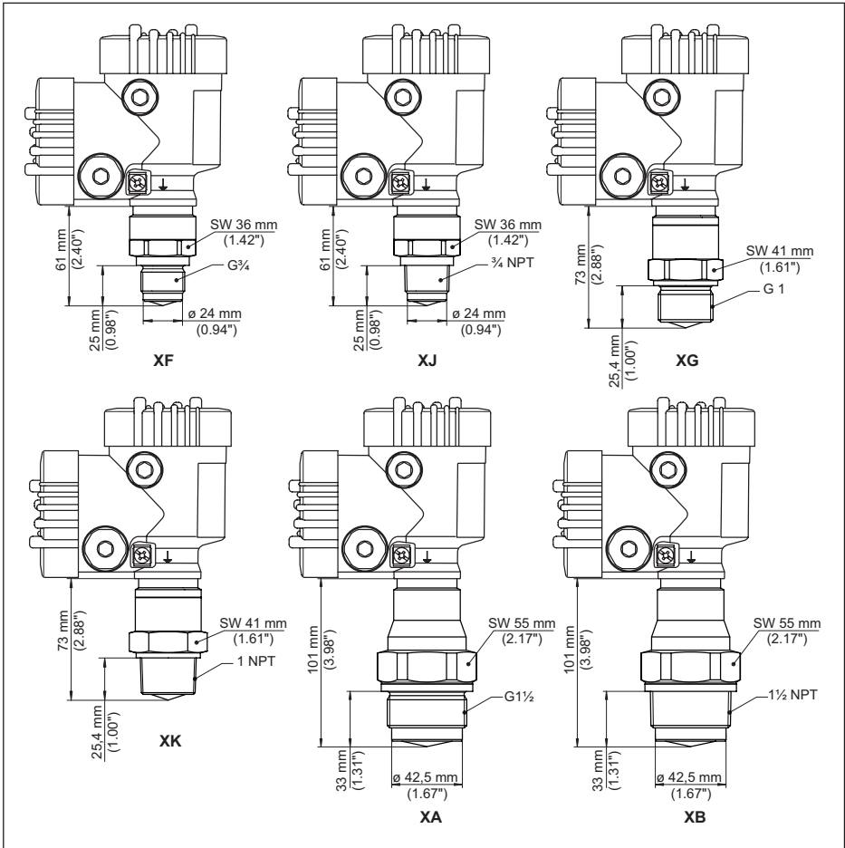
Abb. 86: VEGAPULS 6X, Gewinde mit integriertem Antennensystem bis +150 °C (+302 °F)
