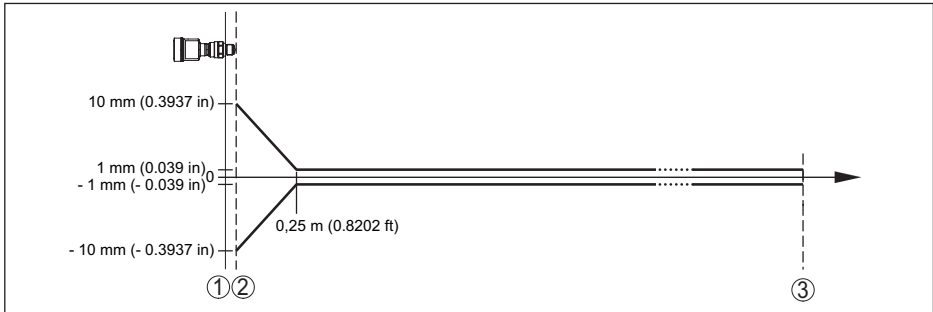
Abb. 63: Messabweichung unter Referenzbedingungen (Beispiel Gewinde mit integriertem Antennensystem, gilt entsprechend für alle Ausführungen) 25)
