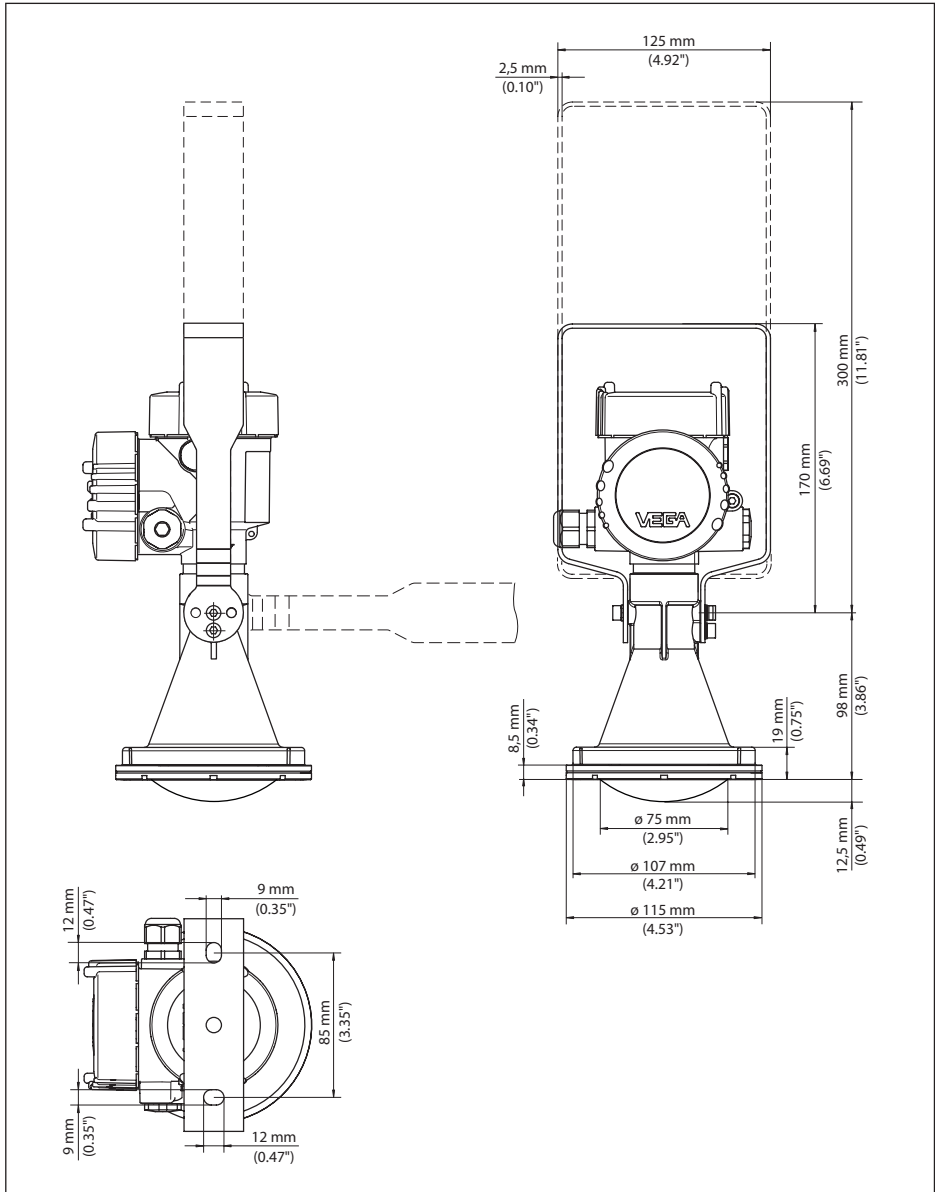
Abb. 84: VEGAPULS 6X, Kunststoff-Hornantenne, Montagebügel in 170 oder 300 mm Länge
