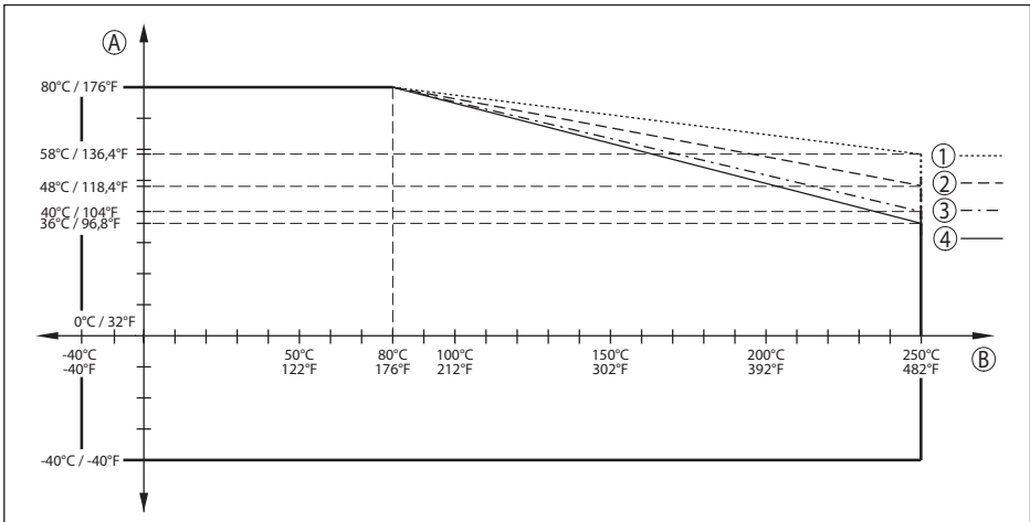
Abb. 67: Derating Umgebungstemperatur, Gewinde mit integriertem Antennensystem bis +250 °C (+482 °F)
