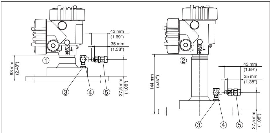
Abb. 97: VEGAPULS 6X, Flansch mit Linsenantenne und Spülluftanschluss
