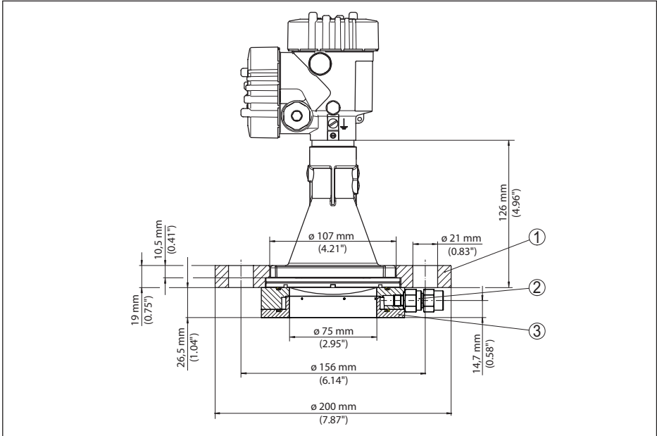
Abb. 81: VEGAPULS 6X mit Überwurfflansch und Spülluftanschluss passend für 3" 150 lbs, DN 80 PN 16
