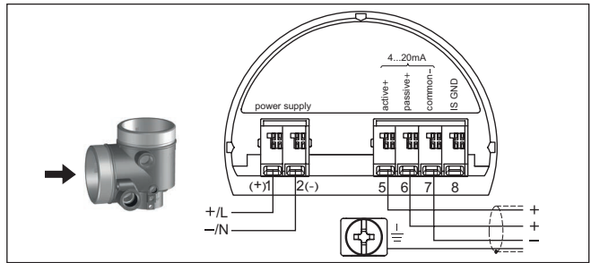
Abb. 46: Anschlussraum Zweikammergehäuse bei Klein- spannung
