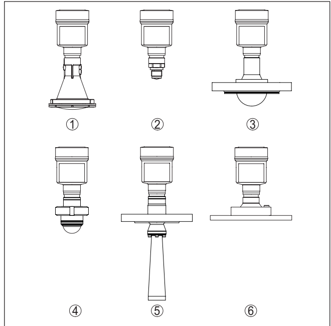
Abb. 1: Antennensysteme VEGAPULS 6X
