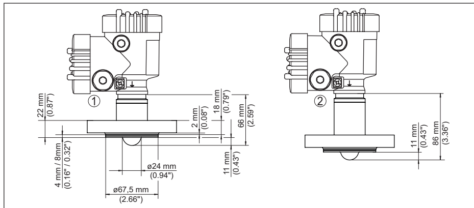
Fig. 91: VEGAPULS 6X, sistema de antena blindado DN 25 PN 40
