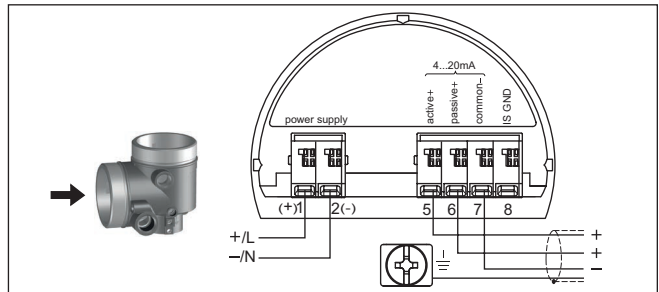
Fig. 46: Compartimento de conexão da caixa e duas câmaras para baixa tensão
