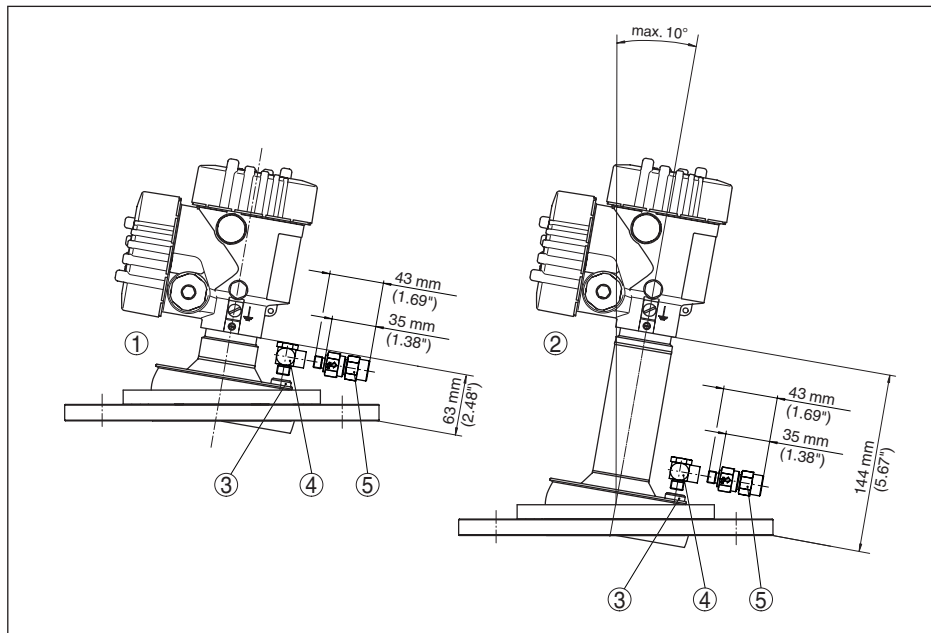
Fig. 99: VEGAPULS 6X, flange com antena lentiforme, suporte giratório e conexão de ar de limpeza
