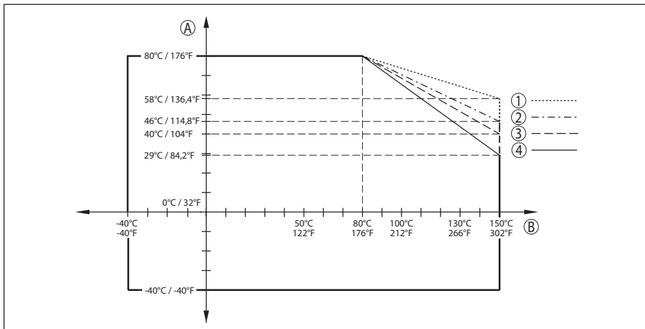
Fig. 76: Redução da temperatura ambiente, flange com antena tipo corneta até +150 °C (+302 °F)
