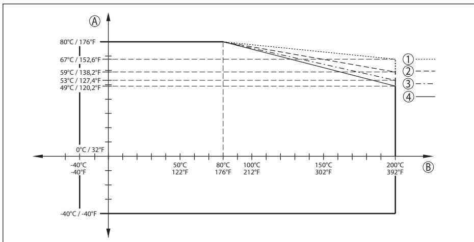
Fig. 77: Redução da temperatura ambiente, flange com antena tipo corneta até +200 °C (+392 °F)
