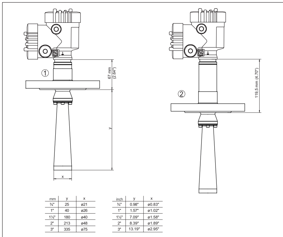
Fig. 88: VEGAPULS 6X, flange com antena tipo corneta até +150 °C (+302 °F)/+250 °C (+482 °F)
