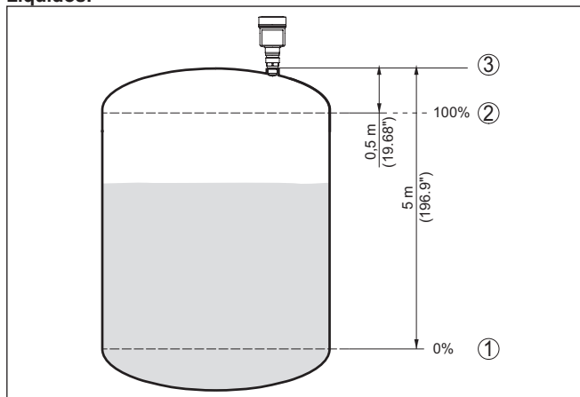
Fig. 50: Exemplo de parametrização calibração de Mín./Máx. - líquidos
