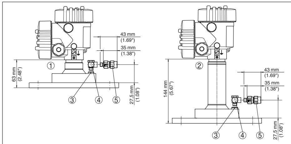
Fig. 97: VEGAPULS 6X, flange com antena lentiforme e conexão de ar de limpeza
