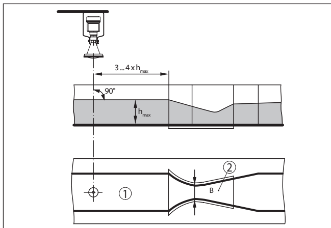
Fig. 43: Medição de débito com calha Venturi Khafagi : h_{\text{máx.}} = enchimento máx. da calha; B = maior estrangulamento da calha
