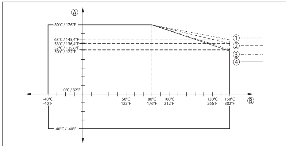
Fig. 72: Redução da temperatura ambiente, flange com antena lentiforme até +150 °C (+302 °F)
