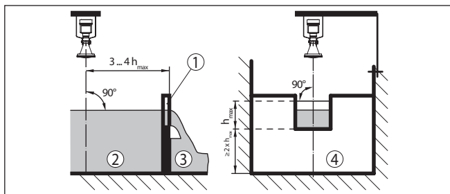
Fig. 42: Medição de débito com vertedouro retangular: h_{\text{máx.}} = \text{máx. enchimento da calha retangular}
