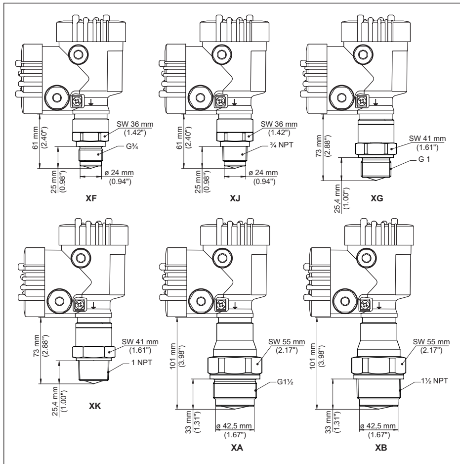
Fig. 86: VEGAPULS 6X, rosca com sistema de antena integrado até +150 °C (+302 °F)
