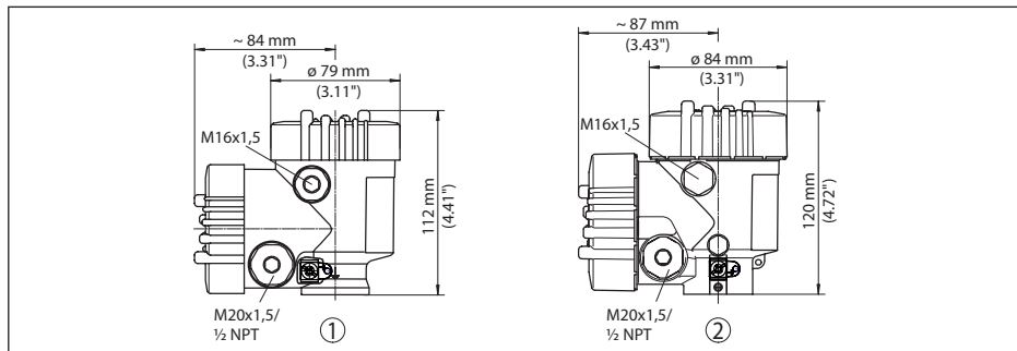
Fig. 79: VEGAPULS 6X; com o módulo de visualização e configuração, a altura da caixa é aumentada em 9 mm (0.35 in)
