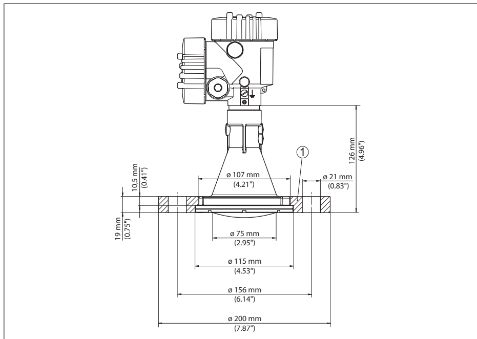
Fig. 80: VEGAPULS 6X com flange de capa adequado para 3" 150 lbs, DN 80 PN 16
