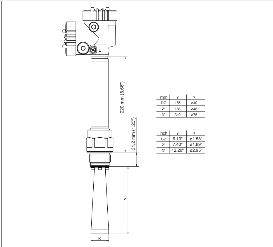
Fig. 89: VEGAPULS 6X, rosca com antena tipo corneta modelo 450 °C
