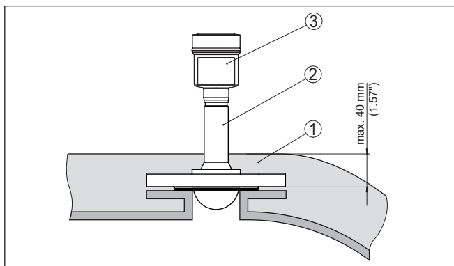
Fig. 28: Montagem do dispositivo em reservatórios isolados
