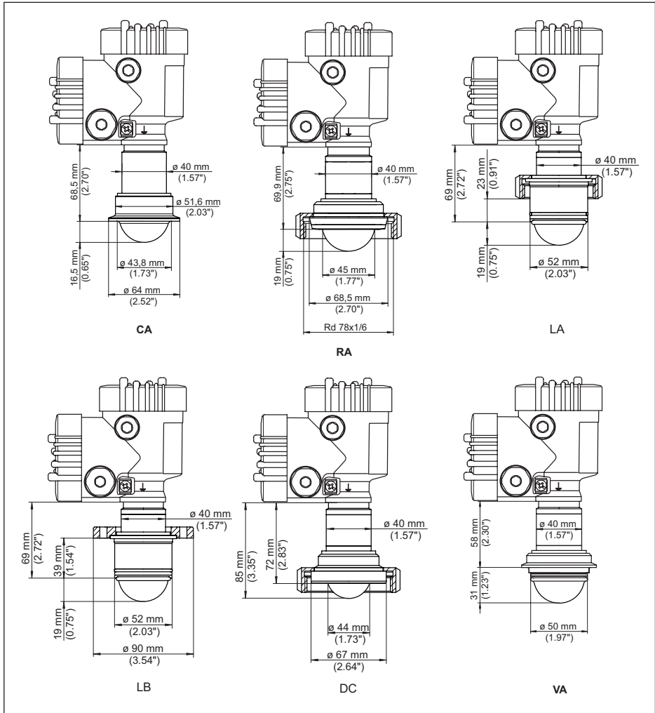
Fig. 94: VEGAPULS 6X, conexão asséptica
