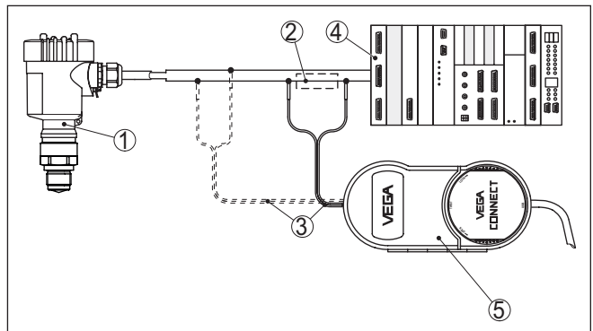
Fig. 3: Conexão do PC à linha de sinais
