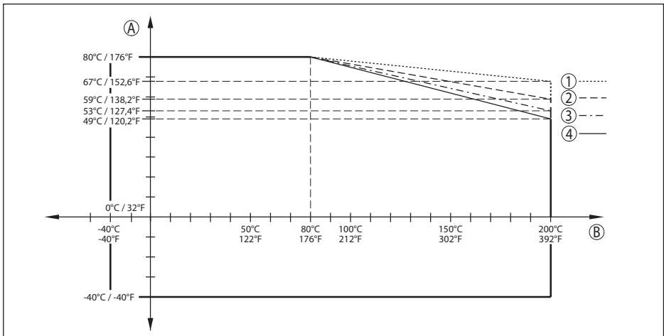
Fig. 66: Redução da temperatura ambiente, rosca com sistema de antena integrado até +200 °C (+392 °F)
