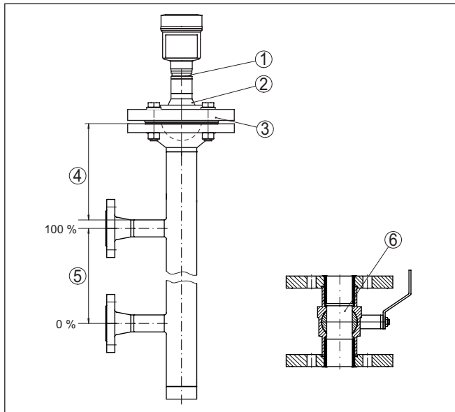
Fig. 41: Estrutura do by-pass
