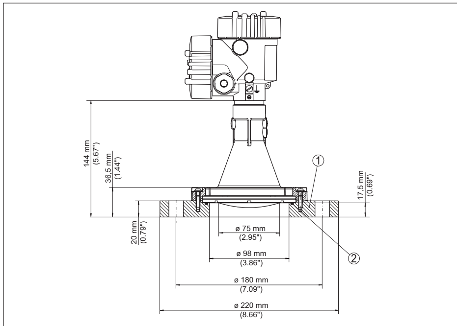
Fig. 82: VEGAPULS 6X com flange adaptador DN 100 PN 6
