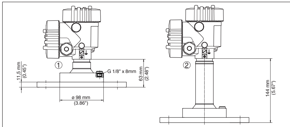
Fig. 96: VEGAPULS 6X, flange com antena lentiforme (espessura da flange, vide desenho, tamanho do flange conforme DIN, ASME, JIS)
