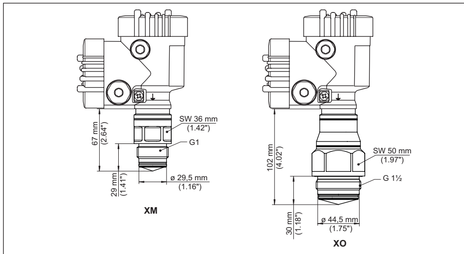
Fig. 93: VEGAPULS 6X, Rosca para adaptador de higiene
