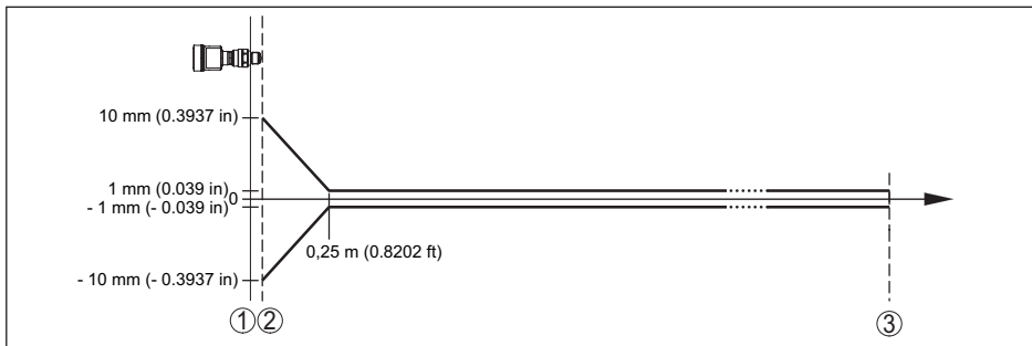
Fig. 63: Diferença de medição sob condições de referência (exemplo: rosca com sistema de antena integrado, vale da mesma forma para todos os modelos) 25)
