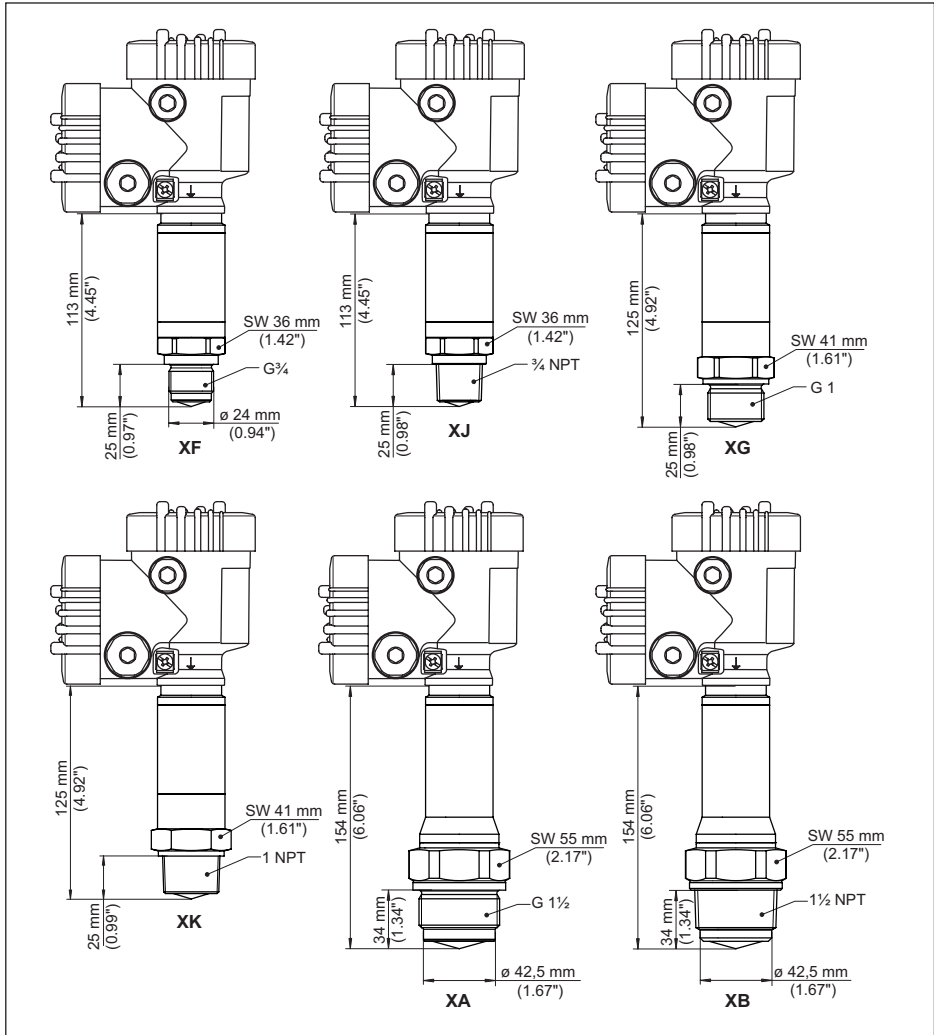
Fig. 87: VEGAPULS 6X, rosca com sistema de antena integrado até +200 °C (+392 °F) e +250 °C (+482 °F)
