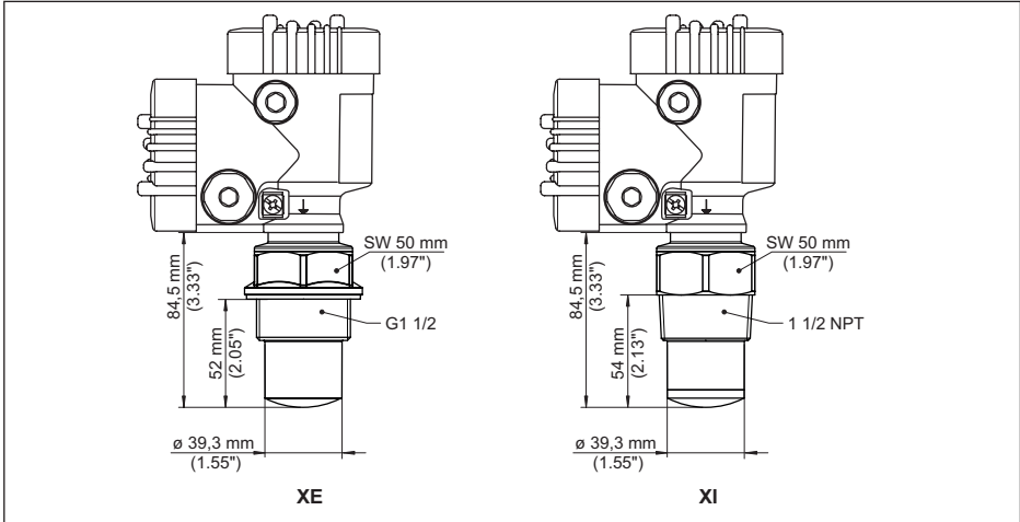
Fig. 85: VEGAPULS 6X, rosca com sistema de antena integrado até +80 °C (+176 °F)
