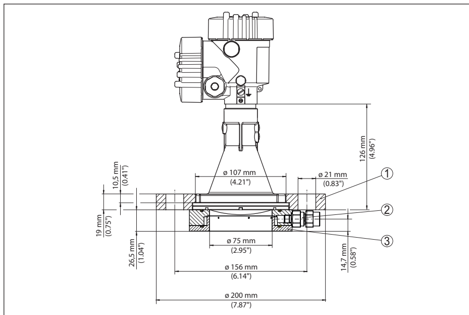
Fig. 81: VEGAPULS 6X com flange de capa e conexão de ar de limpeza adequado para 3" 150 lbs, DN 80 PN 16
