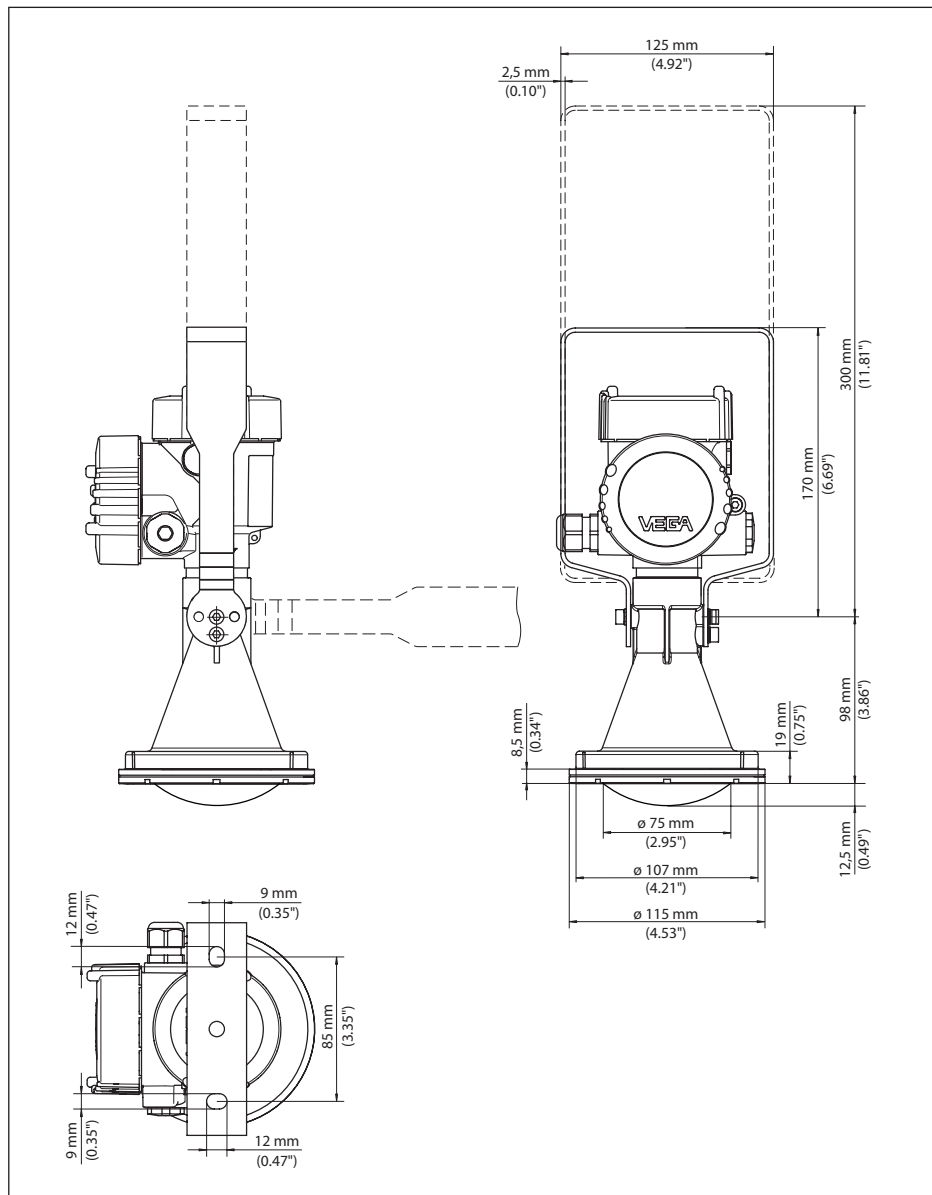
Fig. 84: VEGAPULS 6X, antena de plástico tipo corneta, suporte de montagem com 170 ou 300 mm de comprimento
