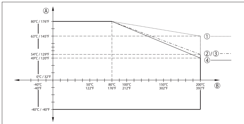
Fig. 73: Redução da temperatura ambiente, flange com antena lentiforme até +200 °C (+392 °F)
