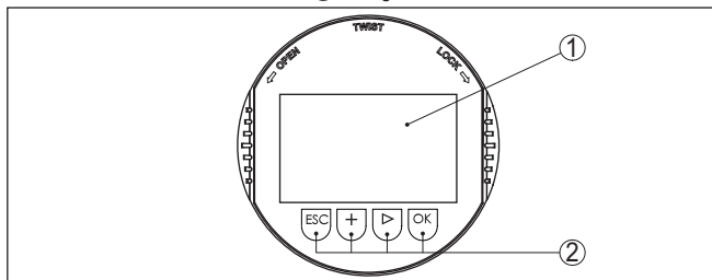
Fig. 48: Elementos de visualização e configuração
