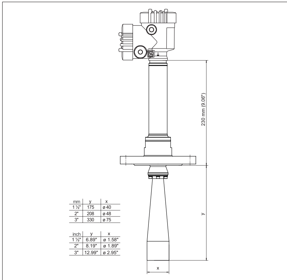
Fig. 90: VEGAPULS 6X, flange com antena tipo corneta modelo 450 °C
