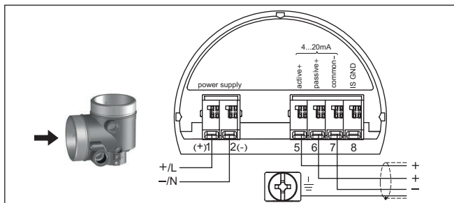
Figura 7: Vano di connessione custodia a due camere per bassa tensione
