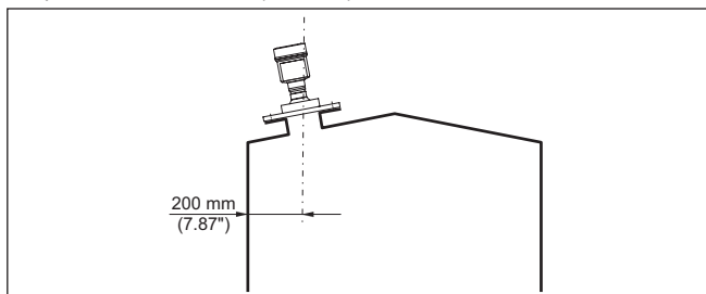
Fig. 4: Montagem do sensor de radar no teto de reservatório
