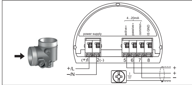
Fig. 7: Compartimento de conexão da caixa e duas câmaras para baixa tensão
