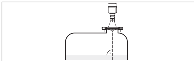
Fig. 12: Uittijnen in vloeistoffen
