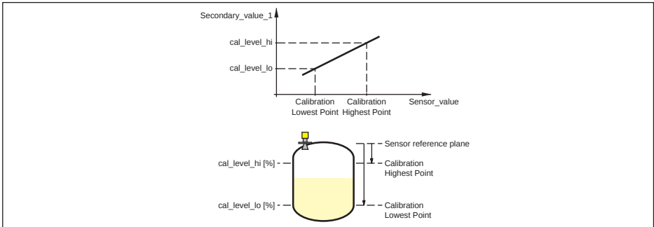
Fig. 43: Inregeling VEGAPULS 61
