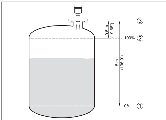
Fig. 34: Parametreervoorbeeld min.-/max.-inregeling
