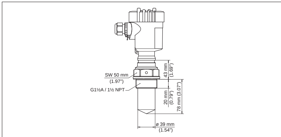
Fig. 49: VEGAPULS 61, schroefdraaduitvoering G1½ , 1½ NPT
