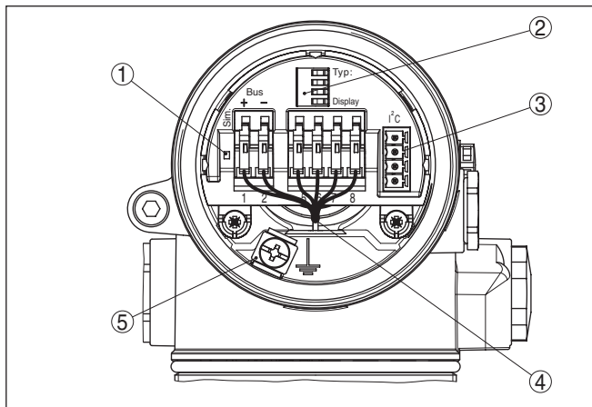
Fig. 28: Elektronicaruimte - tweekamerbehuizing
