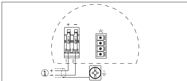
Fig. 26: Aansluitschema - tweekamerbehuizing
