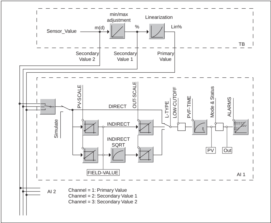
Fig. 42: Meetwaardeverwerking VEGAPULS 61
