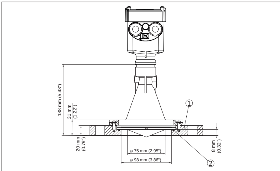
Fig. 53: VEGAPULS 61, adapterflens DN 100, DN 150
