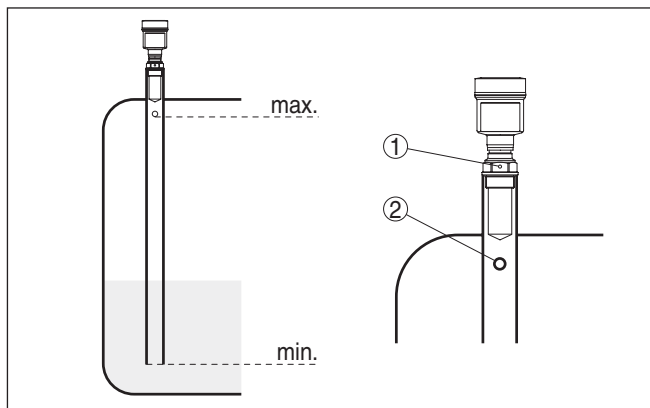
Fig. 15: Pijpantennesystemen in tank. Het ontluchtingsgat in de dippijp moet in hetzelfde vlak als de polarisatiemarkering op de sensor liggen.
