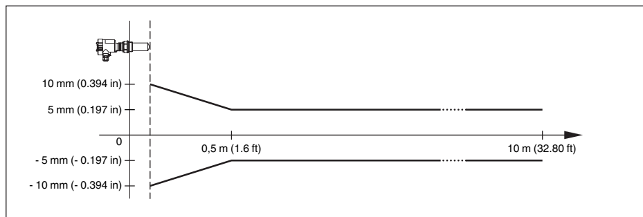
Fig. 38: Meetafwijking VEGAPULS 61 met gekapseld antennesysteem
