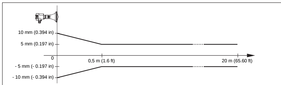
Fig. 40: Meetafwijking VEGAPULS 61 met kunststof hoornantenne
