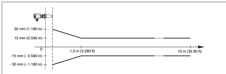
Fig. 39: Meetafwijking VEGAPULS 61 met gekapseld antennesysteem en verhoogde gevoeligheid
