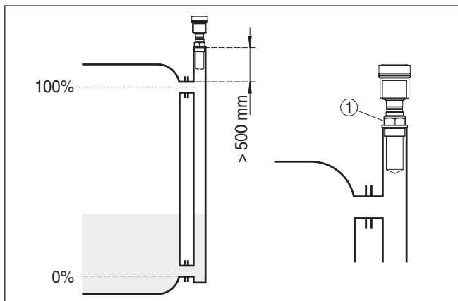
Fig. 16: VEGAPULS 61 in een bypass. De polarisatiemarkering op de procesaansluiting moet in hetzelfde vlak liggen als de pijpgaten of de pijpansluitopeningen.
