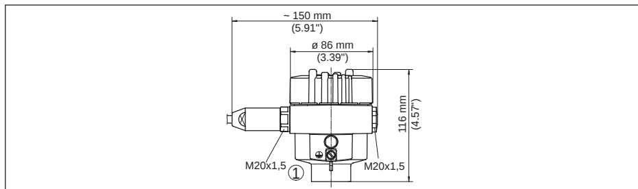
Fig. 46: Huisuitvoeringen in beschermingsklasse IP 66/IP 68, (1 bar), (met ingebouwde display- en bedieningsmodule wordt het huis 18 mm hoger)
