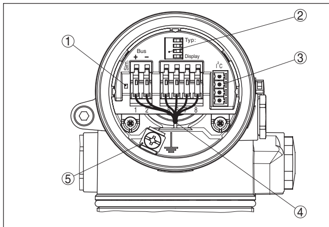
Fig. 24: Elektronicaruimte - tweekamerbehuizing
