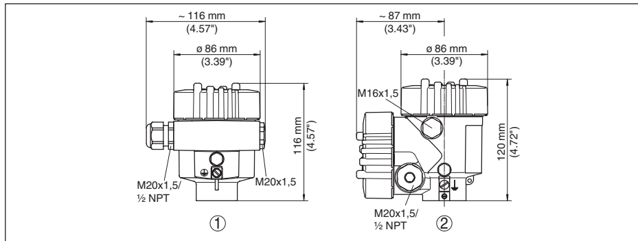
Fig. 45: Huisuitvoeringen in beschermingsklasse IP 66/IP 68, (0,2 bar), (met ingebouwde display- en bedieningsmodule wordt het huis 18 mm hoger)
