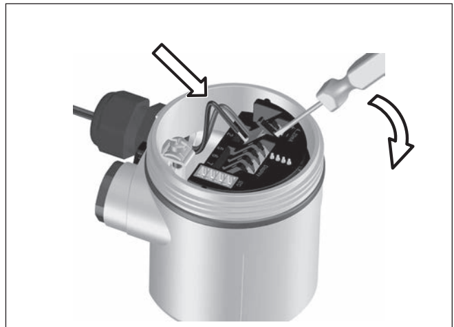
Fig. 19: Aansluitstappen 6 en 7
