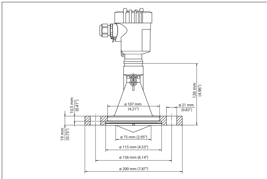
Fig. 52: VEGAPULS 61, overschuifflens DN 80, 3", JIS80
