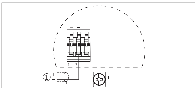
Fig. 30: Aansluitschema Ex-d-ia-tweekamerbehuizing
