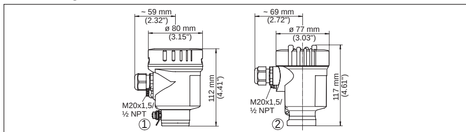
Fig. 47: Huisuitvoeringen in beschermingsklasse IP 66/IP 68, (0,2 bar), (met ingebouwde display- en bedieningsmodule wordt het huis 9 mm/0,35 in hoger, bij positie 1 met 9 mm/0,35 in, bij positie 2 en 3 met 18 mm/0.71 in)
