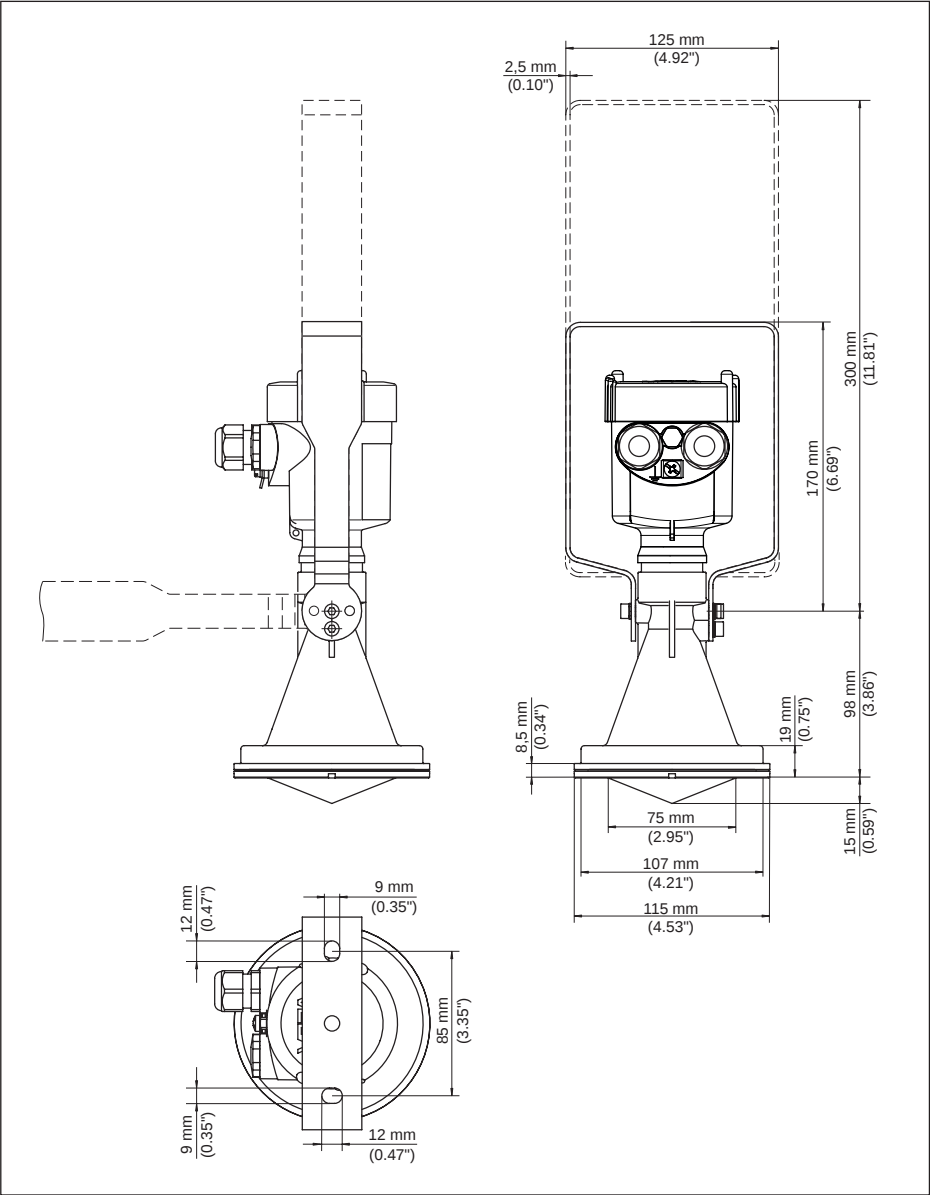
Fig. 51: VEGAPULS 61, uitvoering met montagebeugel in 170 of 300 mm lengte
