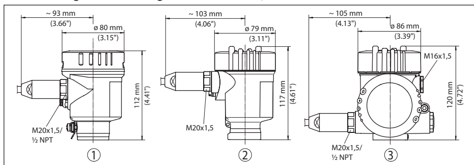
Fig. 48: Huisuitvoeringen in beschermingsklasse IP 66/IP 68, (1 bar), (met ingebouwde display- en bedieningsmodule wordt het huis 18 mm hoger)
