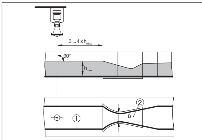
Fig. 18: Flowmetering met Khafagi-venturigoot: d = \text{min. afstand van de sensor} ; h_{\text{max}} = \text{max. vulgraad van de goot} ; B = \text{grootste insnoering van de goot}
