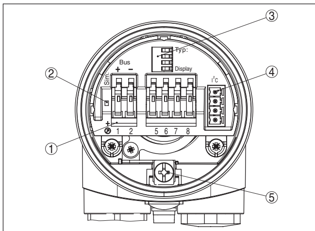
Fig. 21: Elektronica- en aansluitruimte - eenkamerbehuizing
