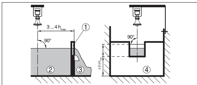
Fig. 17: Flowmetering met rechthoekige overstort: d = \text{min. afstand sensor} ; h_{\text{max}} = \text{max. vulling rechthoekige overstort}
