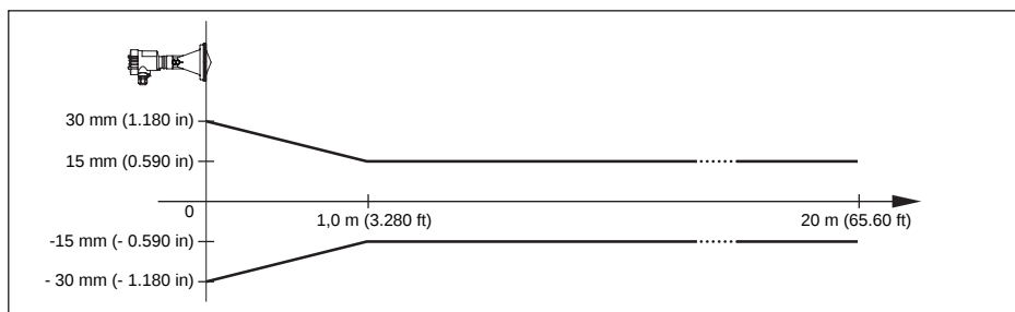
Fig. 41: Meetafwijking VEGAPULS 61 met kunststof hoornantenne en verhoogde gevoeligheid
