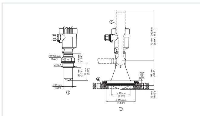
Dimensões VEGAPULS 61
