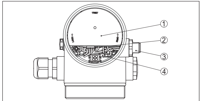
Fig. 29: Vista sobre el compartimiento de la electrónica con adaptados VEGADIS para la conexión de la unidad externa de visualización y configuración
