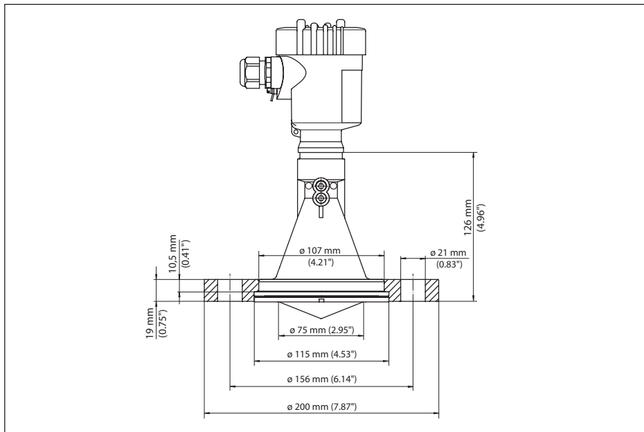
Fig. 68: VEGAPULS 61, brida suelta adecuada para DN 80 PN 16, ASME 3" 150lbs, JIS80 10K
