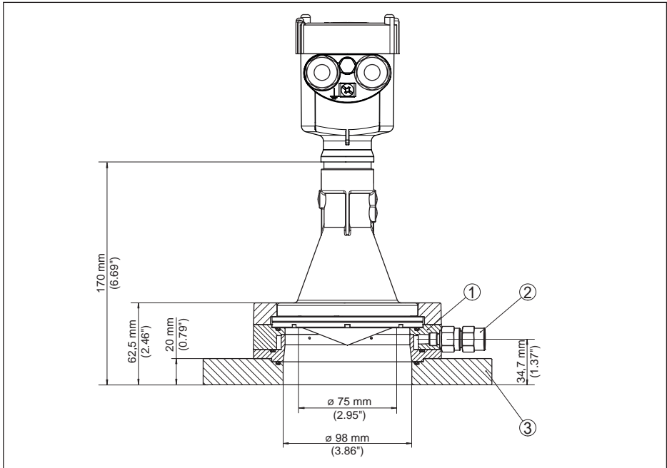
Fig. 71: VEGAPULS 61, brida adaptadora con purga de aire
