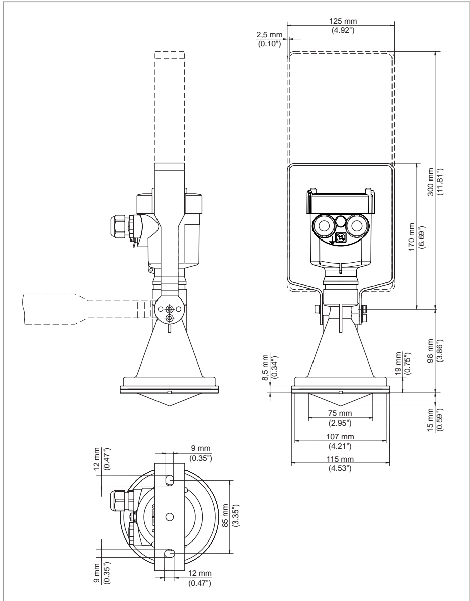
Fig. 65: VEGAPULS 61, estribo de montaje largo 170 o 300 mm
