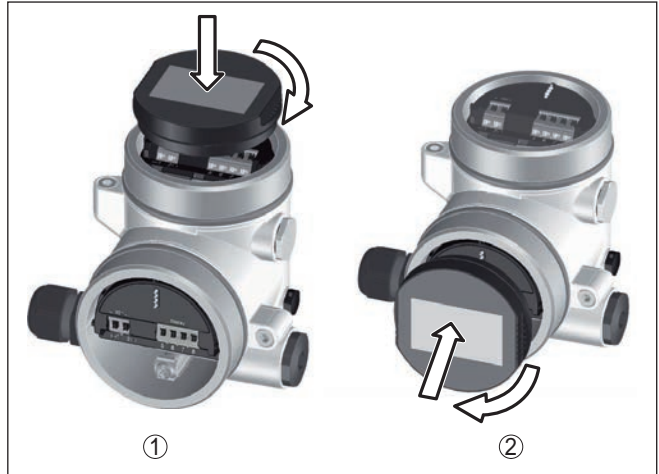
Fig. 33: Empleo del módulo de visualización y configuración en carcasa de dos cámaras
