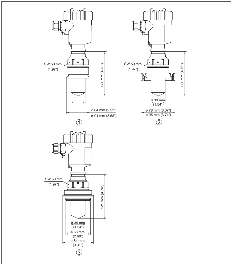
Fig. 64: VEGAPULS 61, conexión aséptica
