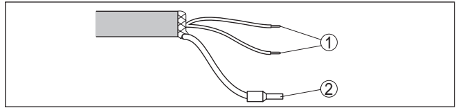
Fig. 31: Dotación de conductores, cable de conexión de conexión fija
