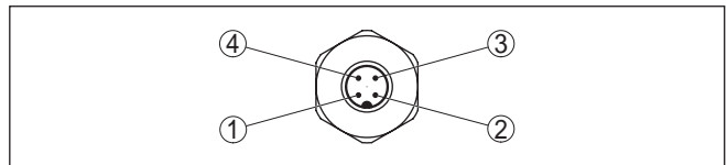
Fig. 28: Vista sobre el conector enchufable
