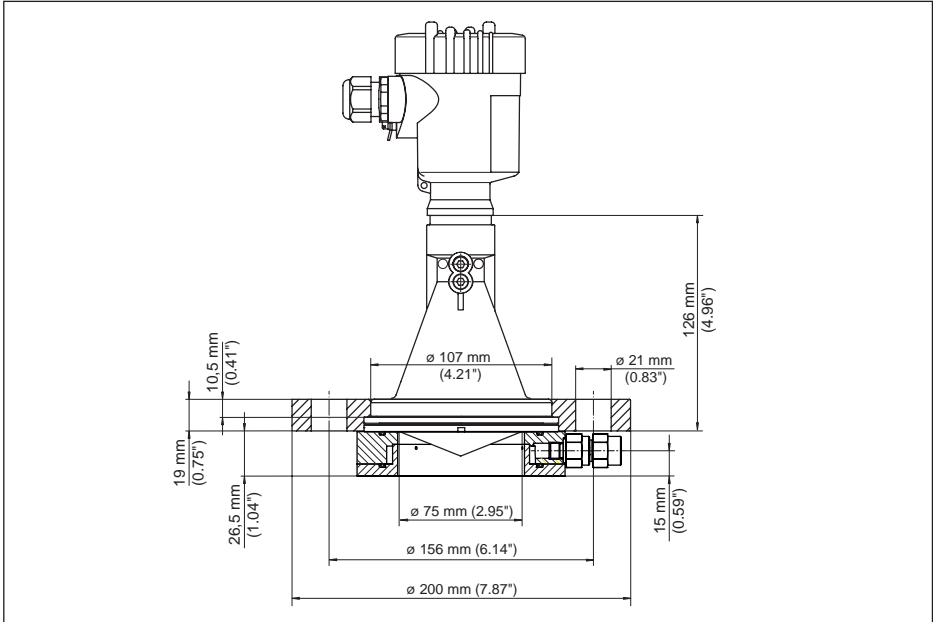
Fig. 69: VEGAPULS 61, brida suelta con conexión de purga, válida para DN 80 PN 16, ASME 3" 150lbs, JIS80 10K
