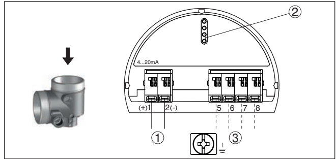
Fig. 26: Compartimiento de la electrónica - Carcasa de dos cámaras Ex-d-ia
