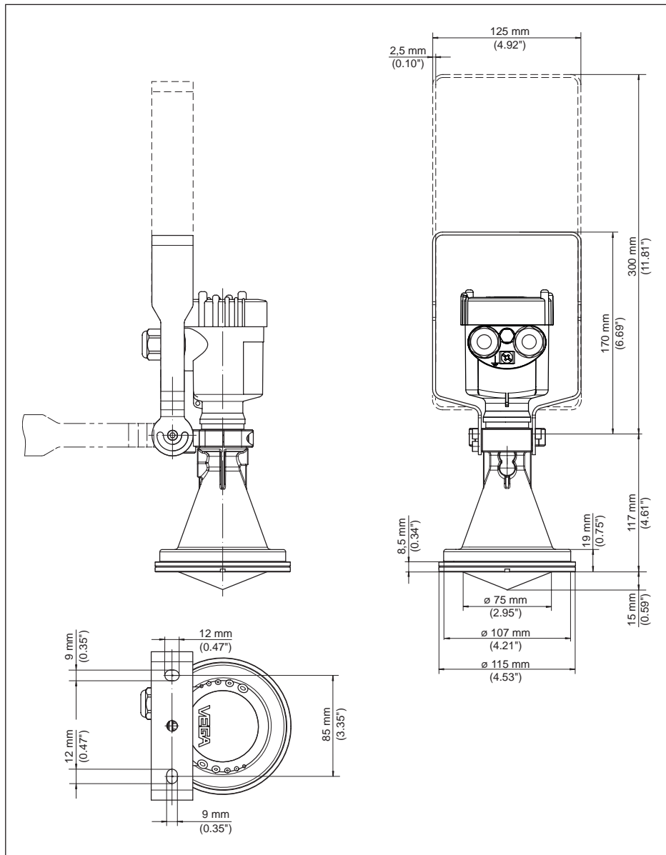
Fig. 66: VEGAPULS 61, estribo de montaje largo 170 o 300 mm
