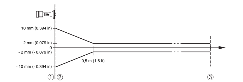
Fig. 57: Error de medición y condiciones de referencia - antena de bocina plástica
