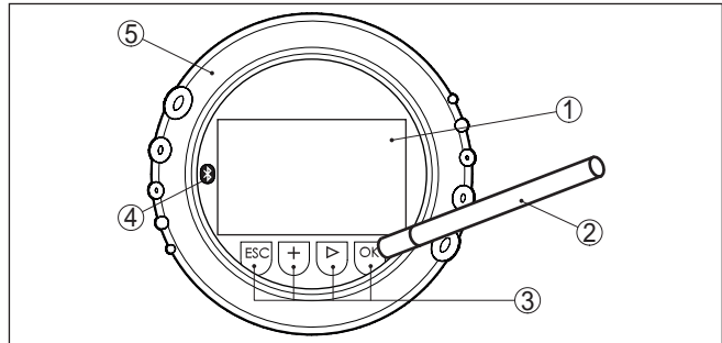
Fig. 35: Elementos de indicación y ajuste - con manejo mediante lápiz magnético
