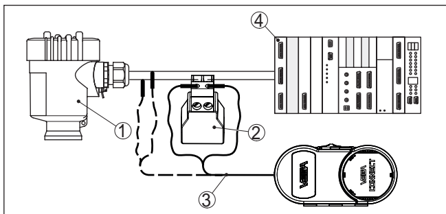
Fig. 38: Conexión del PC a la línea de señal vía HART
