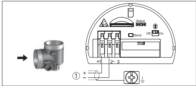
Fig. 25: Compartimiento de conexiones - módulo de radio PLICSMOBILE 81
