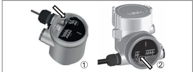
Fig. 21: Pasos de conexión 5 y 6
