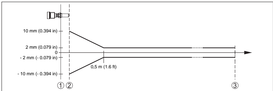
Fig. 56: Error de medición y condiciones de referencia - sistema de antenas encapsulado
