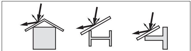
Fig. 14: Tapar los perfiles lisos con pantallas dispersoras
