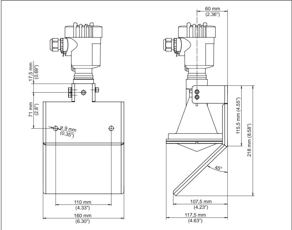
Fig. 67: VEGAPULS 61, soporte de montaje y reflector
