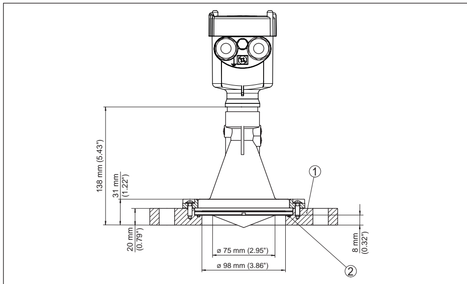
Fig. 70: VEGAPULS 61, brida de adaptación
