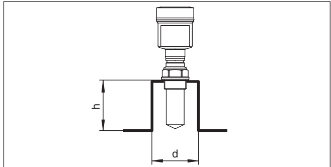
Fig. 10: Medidas diferentes de tubuladuras
