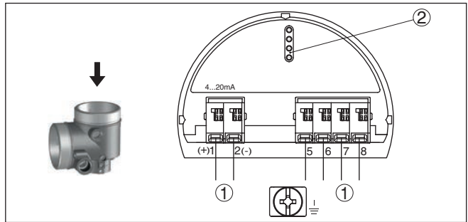
Fig. 23: Compartimento de la electrónica - Carcasa de dos cámaras.
