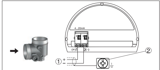
Fig. 27: Compartimiento de conexiones - Carcasa de dos cámaras EX-d-ia
