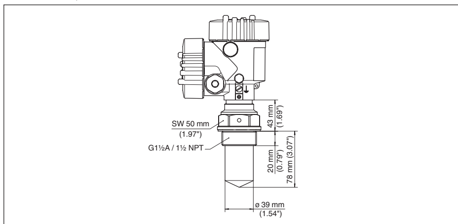
Figura 54: VEGAPULS 61, filettatura G1½, 1½ NPT
