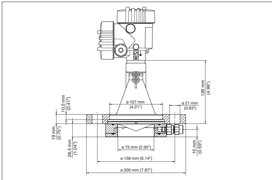
Figura 59: VEGAPULS 61, flangia di raccordo con attacco per spurgo, adeguata a DN 80 PN 16, ASME 3" 150lbs, JIS80 10K
