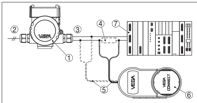
Figura 33: Collegamento del PC via HART alla linea del segnale
