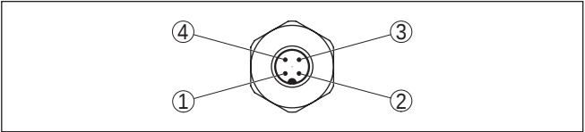
Figura 26: Vista sul connettore a spina M12 x 1
