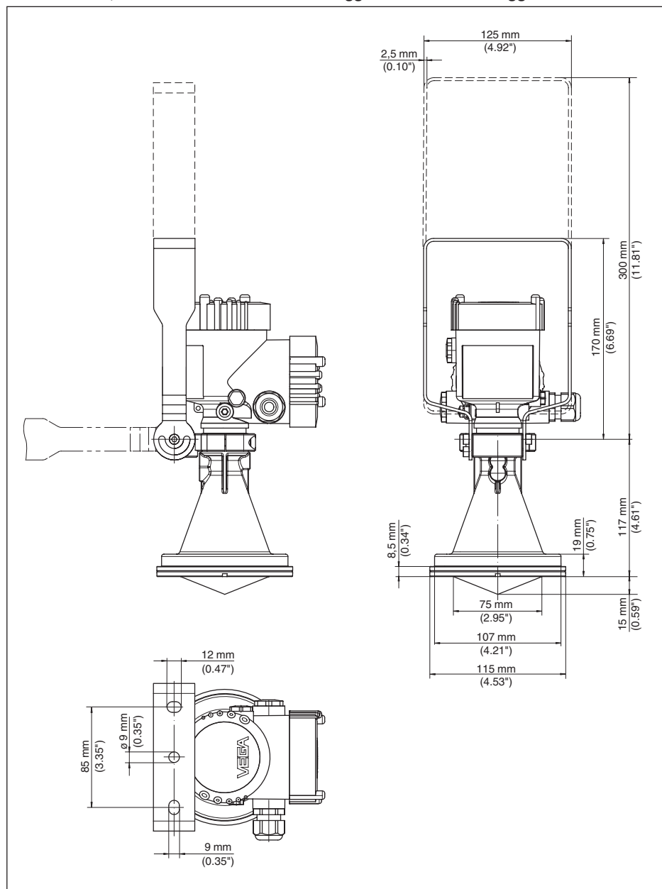
Figura 57: VEGAPULS 61, staffa di montaggio lunga 170 o 300 mm
