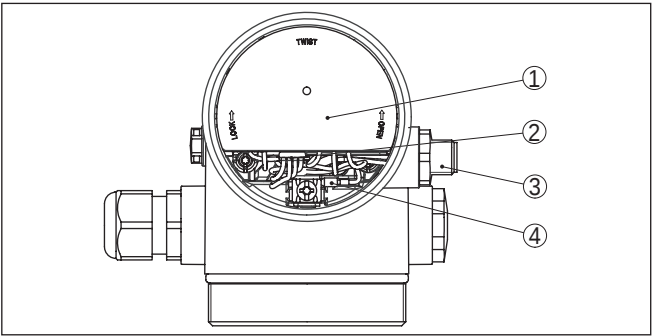
Figura 25: Vista sul vano dell'elettronica con adattatore VEGADIS per il collegamento dell'unità d'indicazione e di calibrazione esterna
