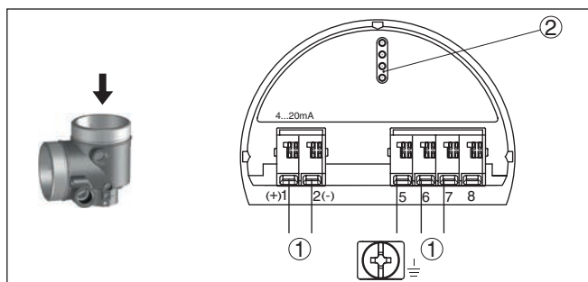
Figura 22: Vano dell'elettronica - custodia a due camere
