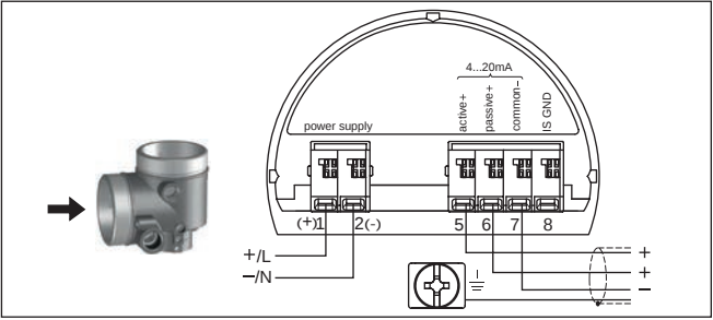
Figura 24: Vano di connessione custodia a due camere per bassa tensione
