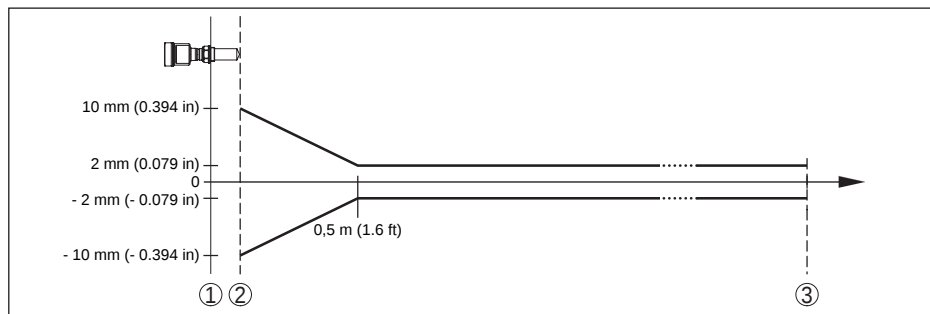
Figura 51: Scostamento di misura sotto condizioni di riferimento - sistema di antenna incapsulata
