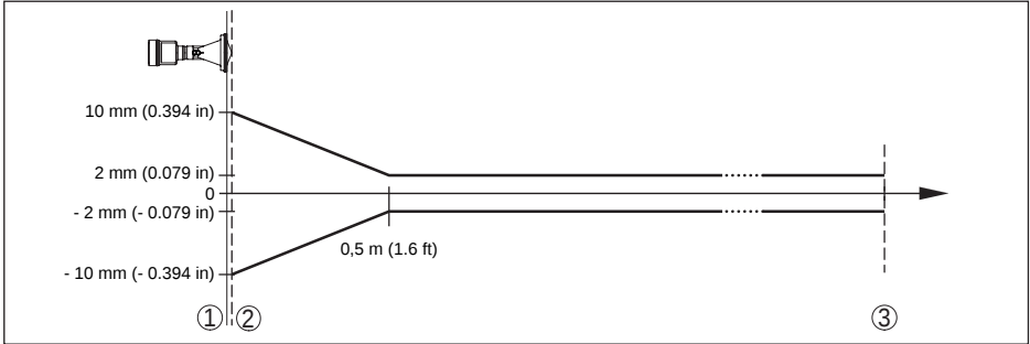
Figura 52: Scostamento di misura in condizioni di riferimento - antenna a cono di resina
