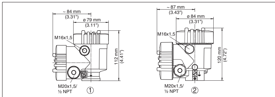
Figura 53: Dimensioni custodia (con tastierino di taratura con display incorporato l'altezza della custodia aumenta di 9 mm/0.35 in, in caso di custodia di metallo di 18 mm/0.71 in)
