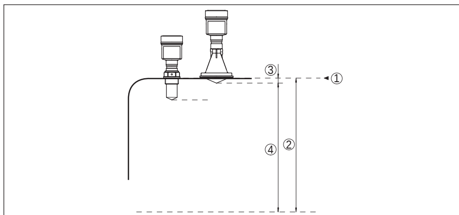
Fig. 50: Data betreffende ingangsgrootte
