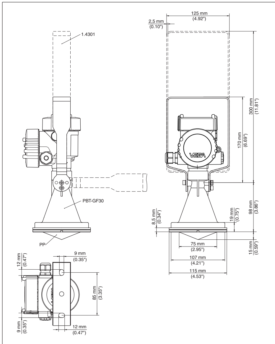
Fig. 56: VEGAPULS 61, montagebeugel in 170 of 300 mm lengte
