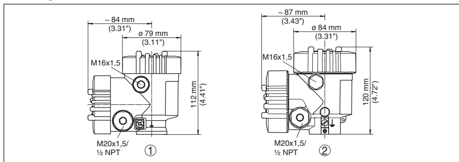
Fig. 53: Afmetingen behuizing (met ingebouwde display- en bedieningsmodule wordt de hoogte van de behuizing 9 mm groter, bij metalen behuizingen 18 mm)
