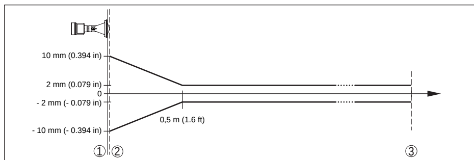
Fig. 52: Meetafwijking onder referentie-omstandigheden - kunststof hoornantenne
