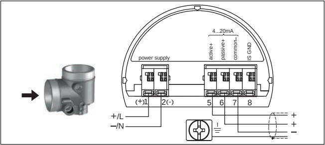
Fig. 24: Aansluitruimte tweekamerbehuizing bij laagspanning
