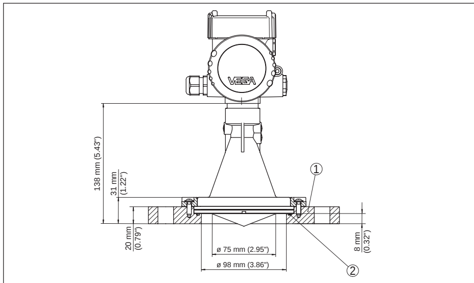
Fig. 60: VEGAPULS 61, adapterflens
