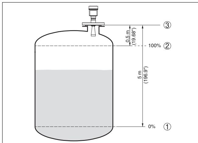
Fig. 31: Parametreevoorbeeld min.-/max.-inregeling
