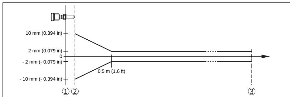
Fig. 51: Meetafwijking onder referentie-omstandigheden - gekapseld antennesysteem
