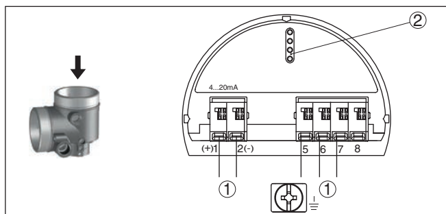
Fig. 22: Elektronicaruimte - tweekamerbehuizing
