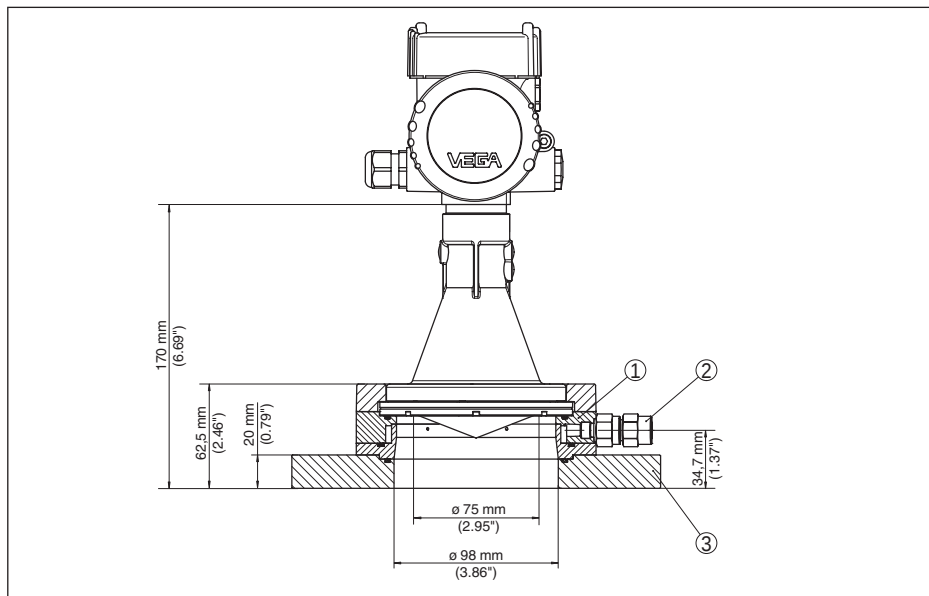
Fig. 61: VEGAPULS 61, adapterflens
