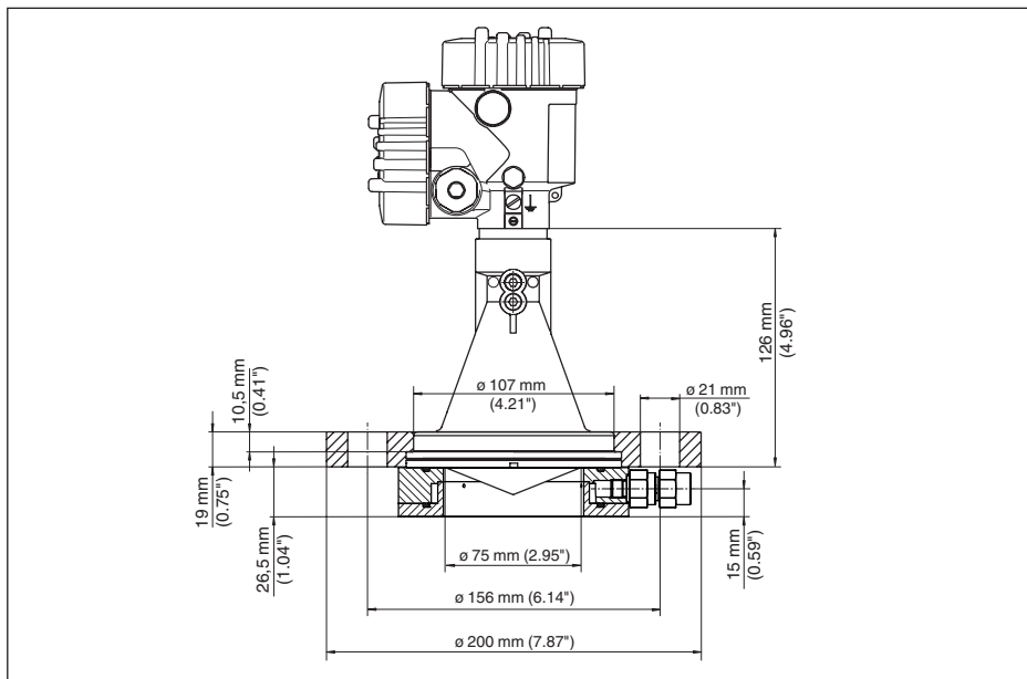
Fig. 59: VEGAPULS 61, overschuifflens met spoelaansluiting, passend voor DN 80 PN 16, ASME 3" 150lbs, JIS80 10K
