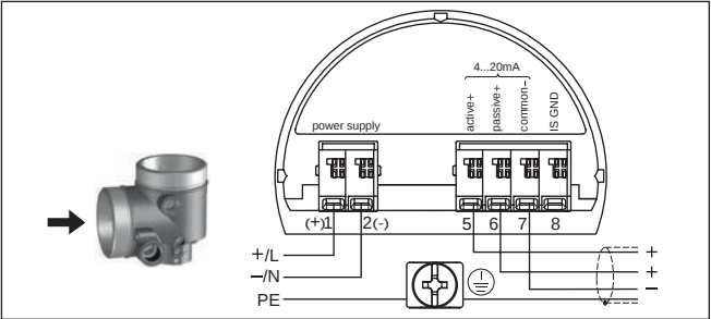
Fig. 23: Aansluitruimte tweekamerbehuizing bij netspanning
