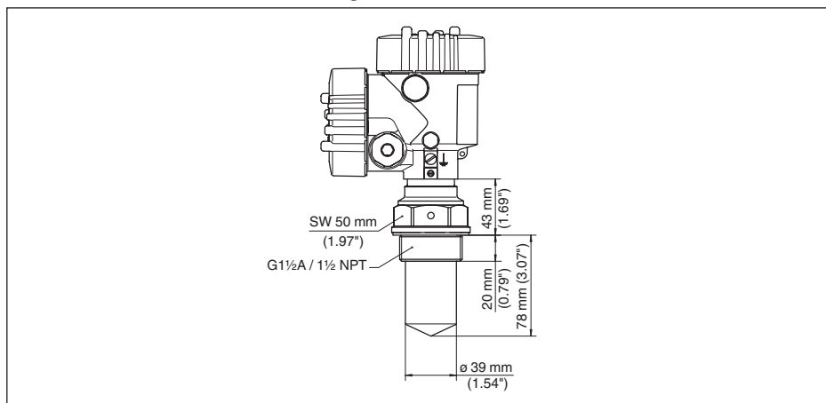
Fig. 54: VEGAPULS 61, schroefdraad G1 1/2, 1 1/2 NPT
