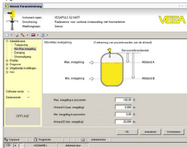
Fig. 34: Voorbeeld van een DTM-aanzicht
