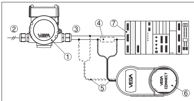
Fig. 33: Aansluiting van de PC via HART op de signaalkabel
