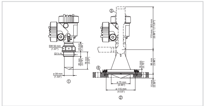
Dimensioni VEGAPULS 61
