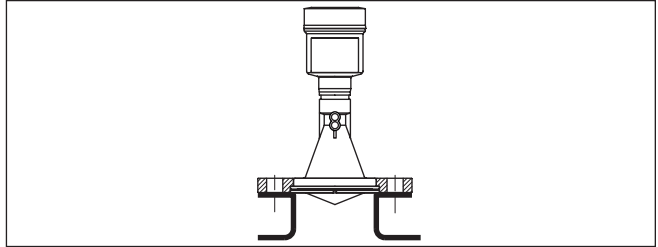
Fig. 9: Montage sur rehausse recommandé
