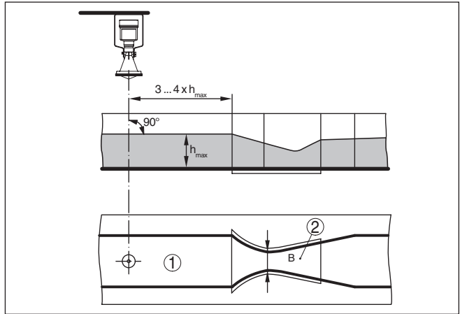
Fig. 18: Mesure du débit avec canal Venturi Khafagi : h_{max} = remplissage max. du canal ; B = resserrement max. du canal
