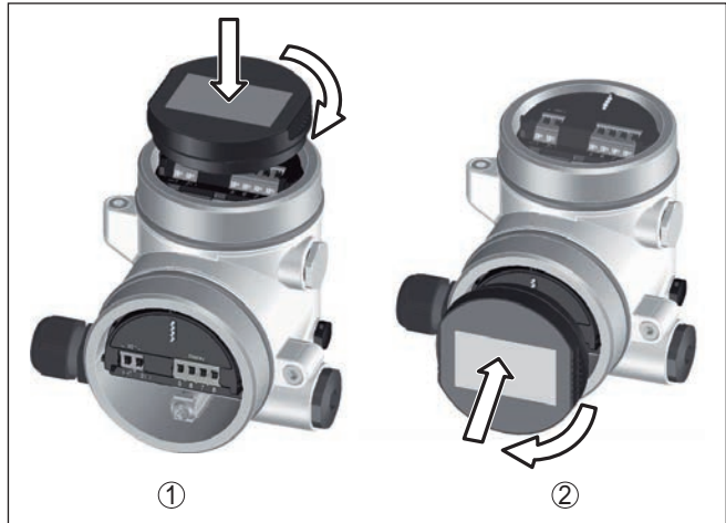
Fig. 26: Montage du module d'affichage et de réglage dans le boîtier à deux chambres
