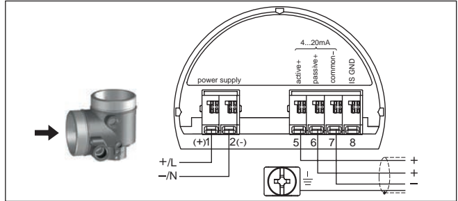
Fig. 22: Compartiment de raccordement boîtier deux chambres pour très basse tension
