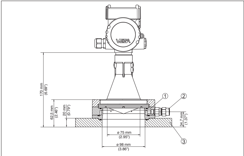
Fig. 55: VEGAPULS 61, bride d'adaptation
