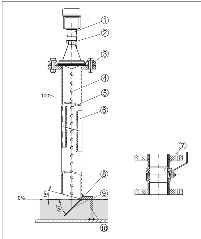
Fig. 14: Structure d'un tube tranquillisateur VEGAPULS 61
