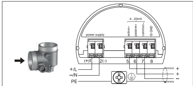
Fig. 21: Compartiment de raccordement boîtier deux chambres pour tension de réseau
