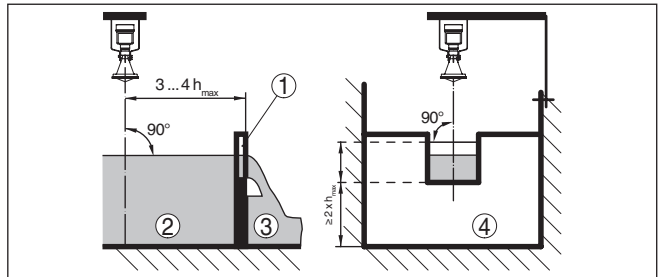
Fig. 17: Mesure de débit avec déversoir rectangulaire : d_{min} = écart minimum du capteur (voir chapitre "Caractéristiques techniques") ; h_{max} = remplissage max. du déversoir rectangulaire
