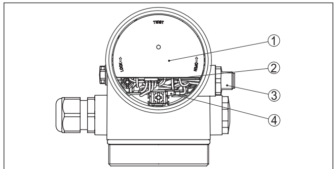
Fig. 23: Vue sur le compartiment de l'électronique avec l'adaptateur VEGADIS pour le raccordement de l'unité de réglage et d'affichage
