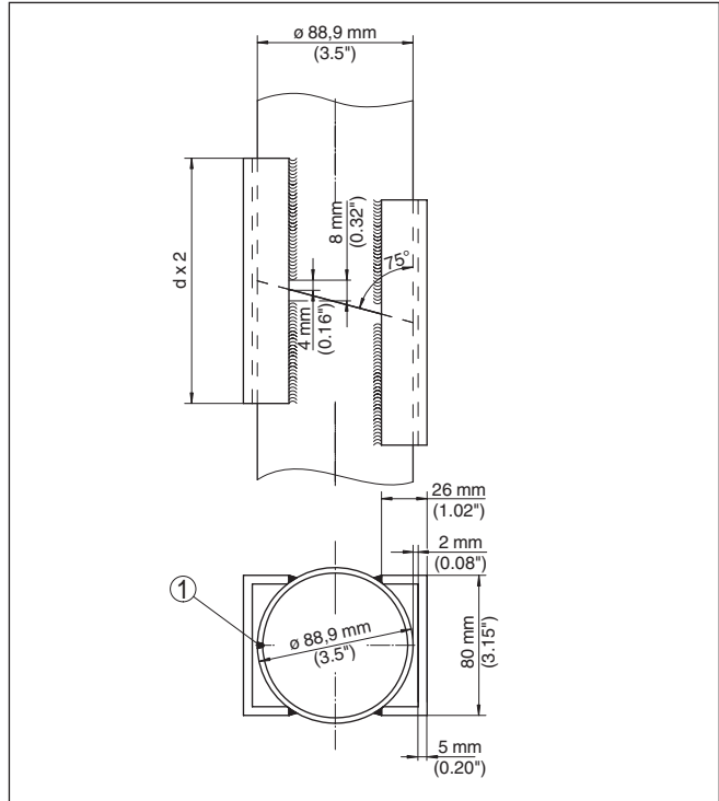
Fig. 15: Soudure sur prolongation de tube tranquillisateur pour différents exemples de diamètres
