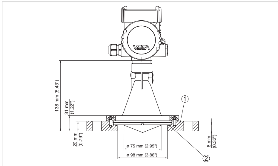
Fig. 54: VEGAPULS 61, bride d'adaptation
