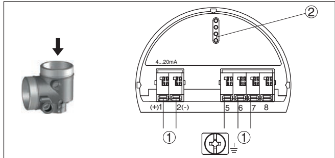
Fig. 20: Compartiment électronique - boîtier à deux chambres
