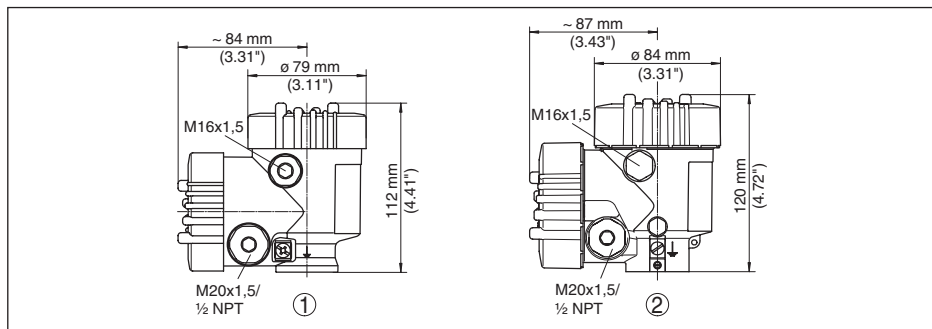
Fig. 50: Cotes du boîtier (avec module de réglage et d'affichage intégré, la taille du boîtier augmente de 9 mm/0.35 in, dans le cas des boîtiers métalliques de 18 mm/0.71 in)
