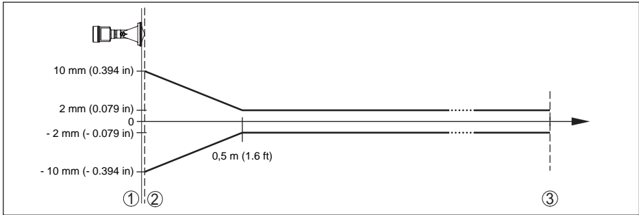
Fig. 49: Écart de mesure sous conditions de référence - antenne cône en plastique
