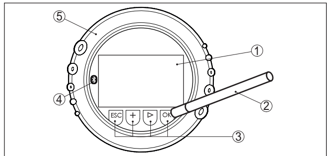
Fig. 28: Éléments de réglage et d'affichage - avec paramétrage par le stylet
