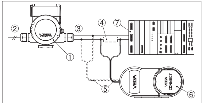
Fig. 31: Raccordement du PC à la ligne signal via HART
