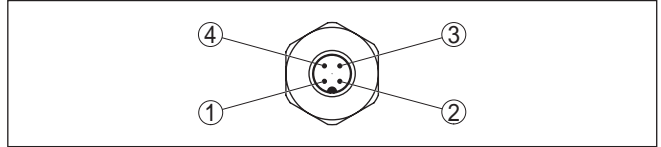
Res. 27: M12 x 1 elektrik bağlantısına bakış
