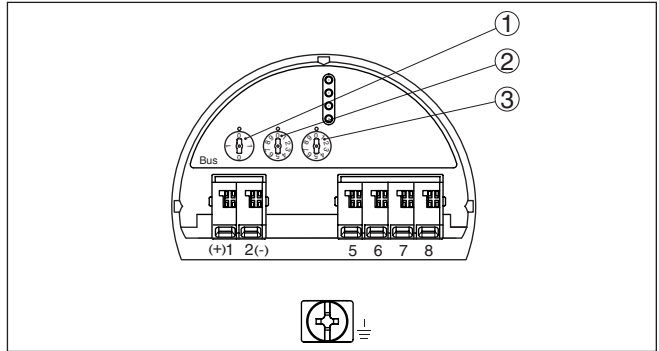
Res. 29: Adres seçme anahtarları
