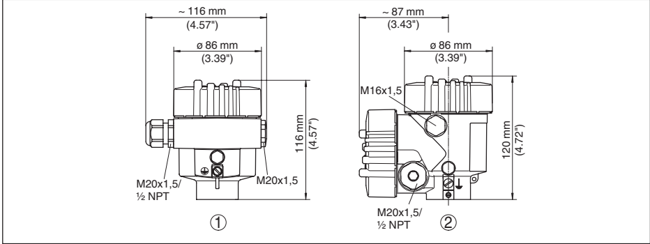
Res. 58: Koruma sınıfı IP 66/IP 68 (0,2 bar) olan gövde modelleri; entegre gösterge ve ayar modülü gövde yüksekliğini 18 mm/0.71 in kadar artırır
