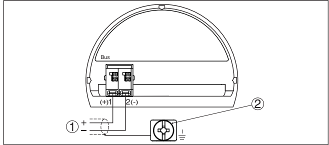
Res. 24: Ex-d-ia iki hücreli gövde - bağlantı bölümü
