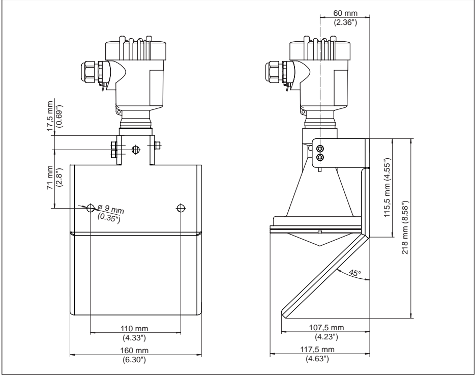
Res. 63: VEGAPULS 61, Montaj kulbu ve reflektör
