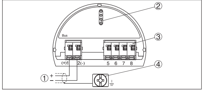
Res. 22: İki hücreli gövde - bağlantı bölmesi
