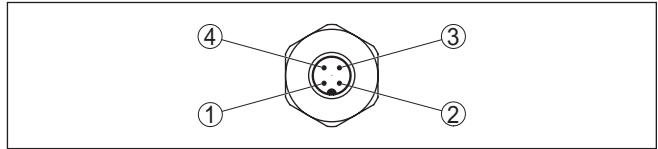
Res. 25: Bağlantı fişine bakış
