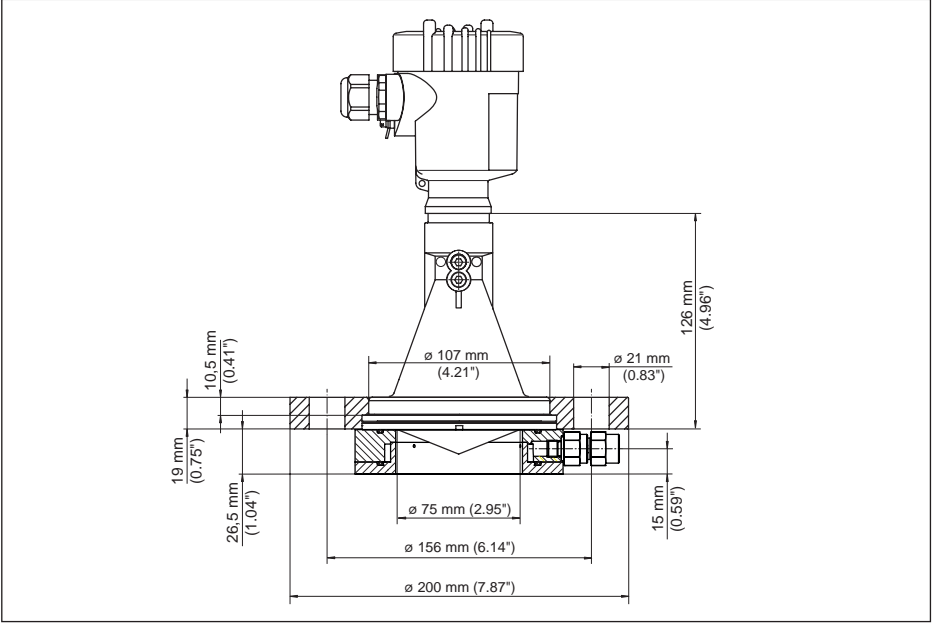
Res. 65: VEGAPULS 61, hava temizlemeli sıkıştırma flanşı, DN 80 PN 16, ASME 3" gereğince 150lbs, JIS80 10K
