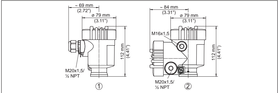
Res. 57: IP 66/IP 67 koruma tipli gövde modelleri (Entegre gösterge ve ayar modülü gövde yüksekliğini 9 mm/0.35 in artırır.)
