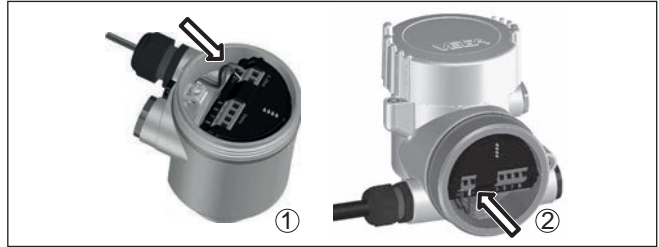
Res. 19: Bağlantı prosedürü 5 ve 6
