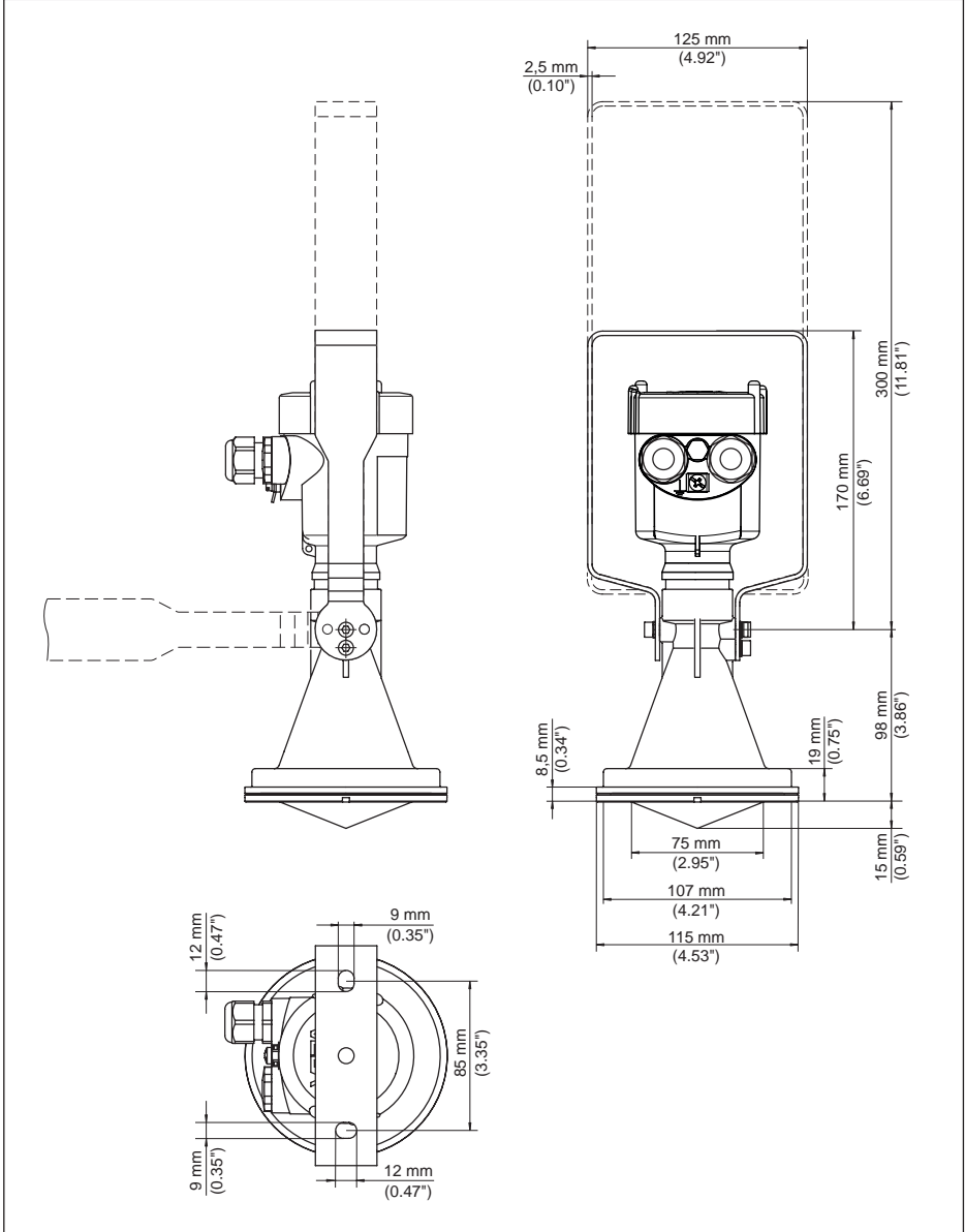
Res. 62: VEGAPULS 61, 170 veya 300 mm uzunluğunda montaj kulbu
