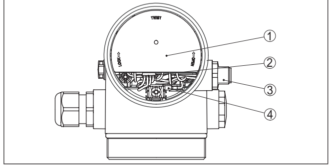
Res. 26: Dış gösterge ve ayar biriminin bağlanması için VEGDIS adaptörlü elektronik bölümüne bakış
