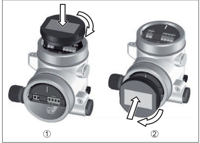
Res. 31: Gösterge ve ayar modülünün iki hücreli gövdeye montajı
