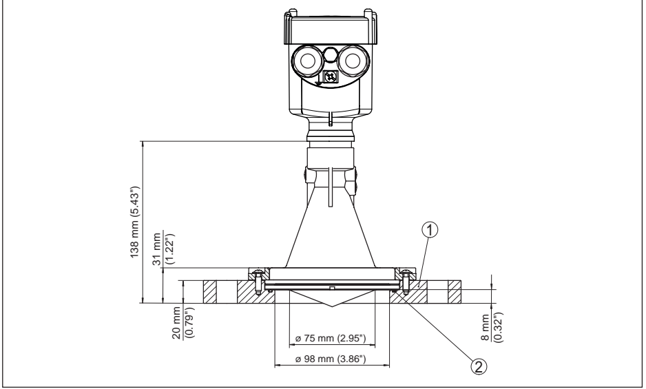
Res. 66: VEGAPULS 61, Adaptör flanş
