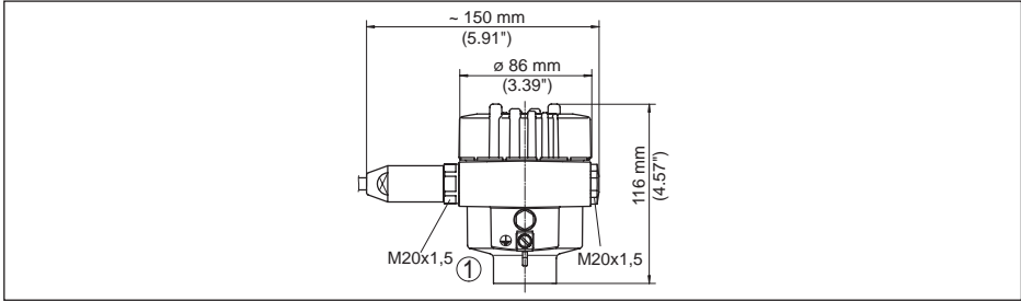
Res. 59: Koruma sınıfı IP 66/IP 68 (1 bar) olan gövde modelleri; (entegre gösterge ve ayar modülü gövde yüksekliğini 18 mm/0.71 in kadar artırır)
