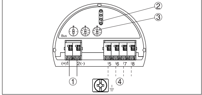
Res. 23: Elektronik bölümü - Ex-d-ia iki hücreli gövde
