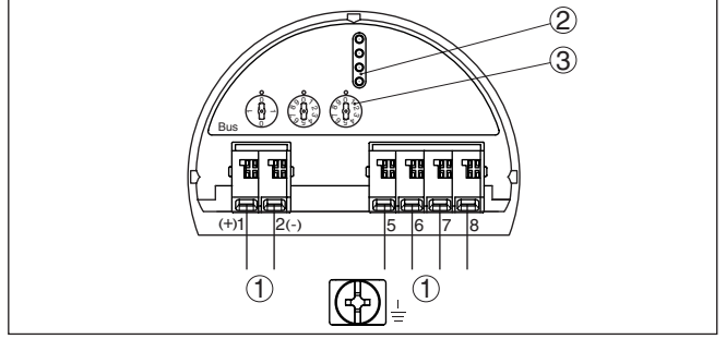
Res. 21: Elektronik bölmesi - iki hücreli gövde
