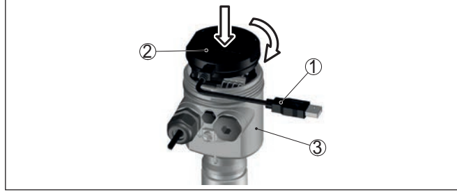
Res. 35: Bilgisayarın arayüz adaptörüyle sensöre doğrudan bağlanması
