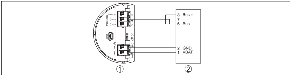
Fig. 52: Aansluiting van de VEGAPULS 61 op RTU ABB Total Flow
