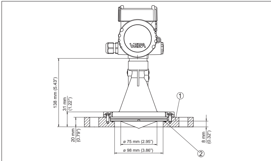
Fig. 60: VEGAPULS 61, adapterflens
