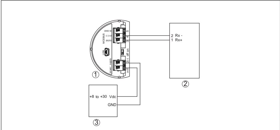
Fig. 53: Aansluiting van de VEGAPULS 61 op de RTU Thermo Electron Autopilot
