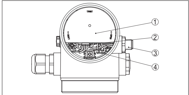
Fig. 23: Een blik op de elektronicarimte met VEGADIS-adapter voor aansluiting van de externe display- en bedieningseenheid
