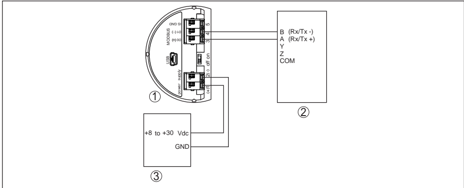
Fig. 51: Aansluiting van de VEGAPULS 61 op RTU Fisher ROC 809
