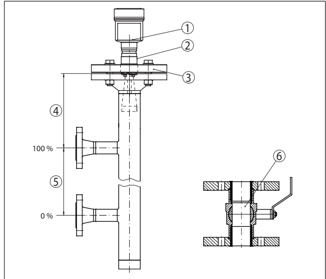
Fig. 16: Opbouw bypass
