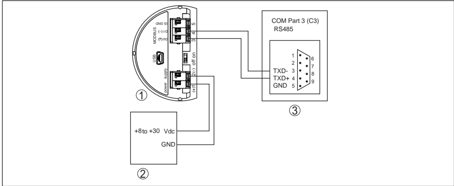
Fig. 55: Aansluiting van de VEGAPULS 61 op RTU ScadaPack
