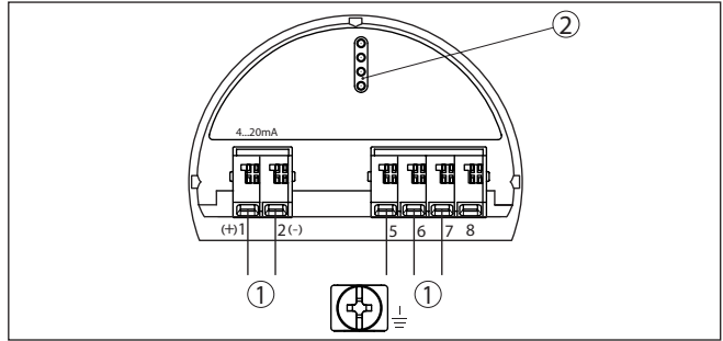
Fig. 21: Elektronicaruimte - tweekamerbehuizing
