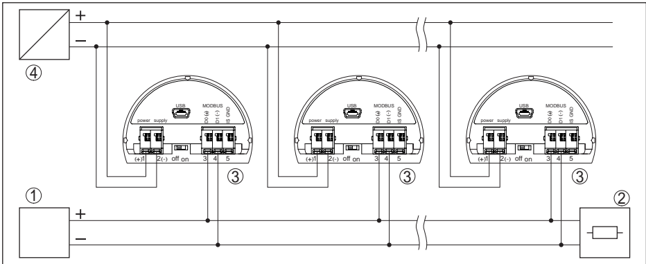
Fig. 50: Busarchitectuur Modbus
