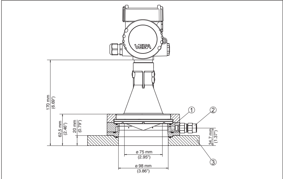
Fig. 61: VEGAPULS 61, adapterflens
