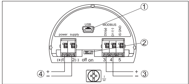
Fig. 22: Aansluitruimte
