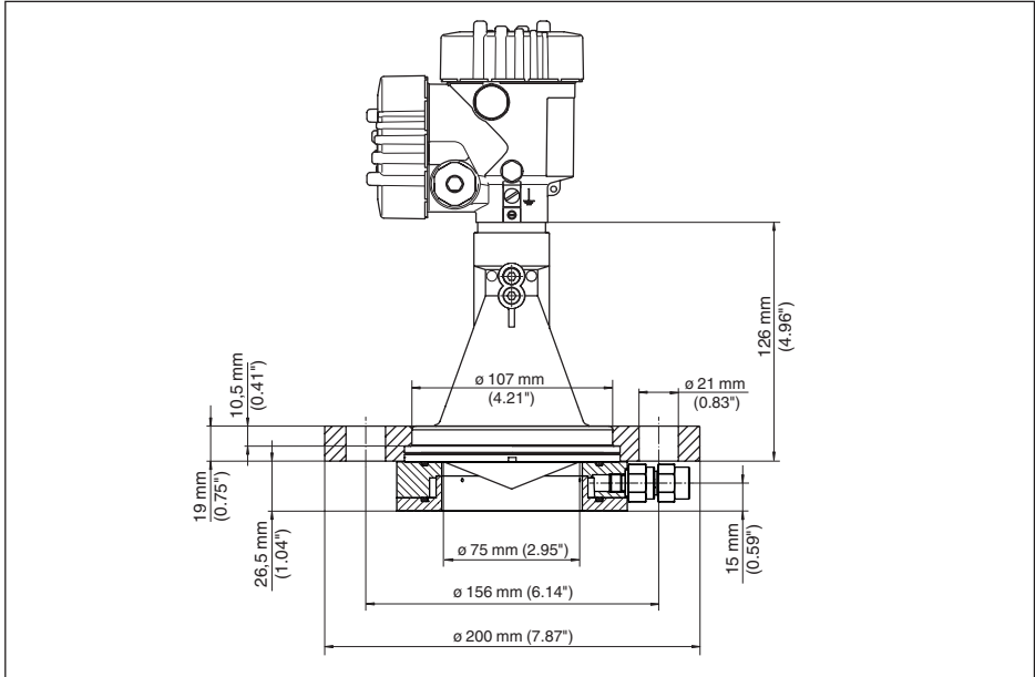
Fig. 59: VEGAPULS 61, overschuifflens met luchtspoeling, passend voor DN 80 PN 16, ASME 3" 150lbs, JIS80 10K
