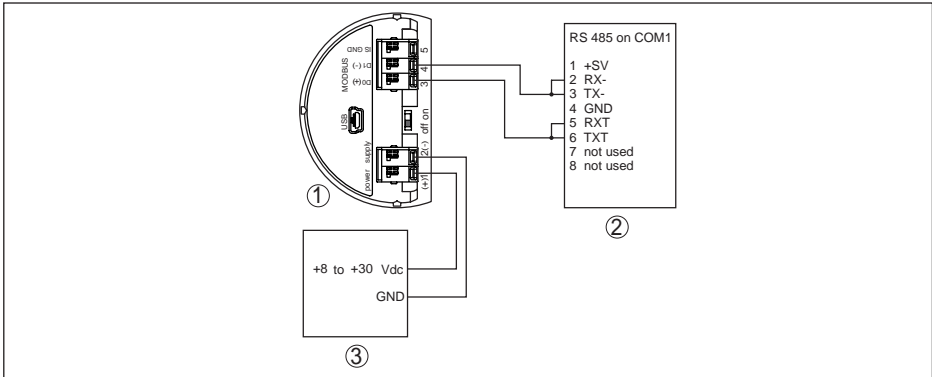
Fig. 54: Aansluiting van de VEGAPULS 61 op de RTU Bristol ControlWave Micro
