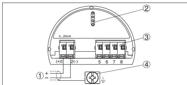
Fig. 7: Elektronica- en aansluitruimte - eenkamerbehuizing
