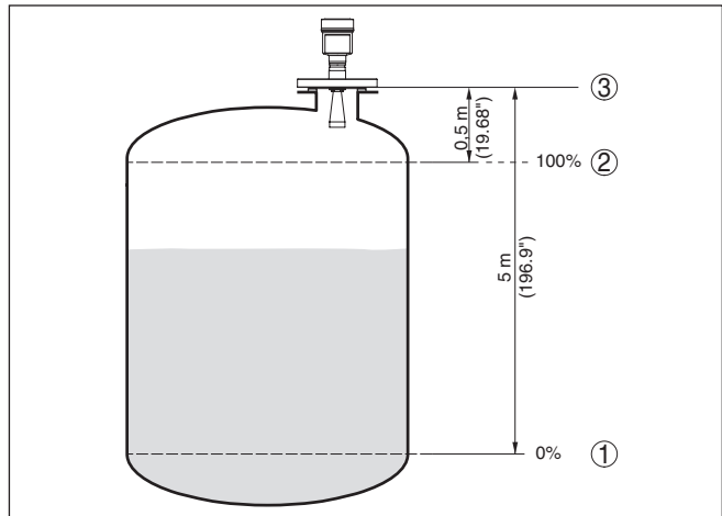
Fig. 11: Parametreervoorbeeld min.-/max.-inregeling
