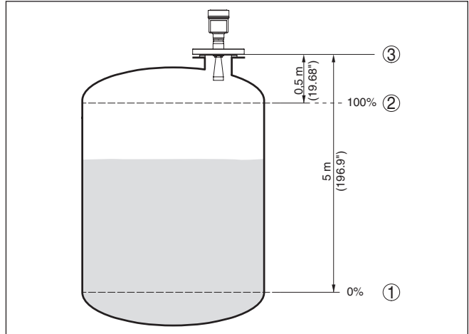
Res. 11: Min./Maks. seviye ayarı parametrelenme örneği
