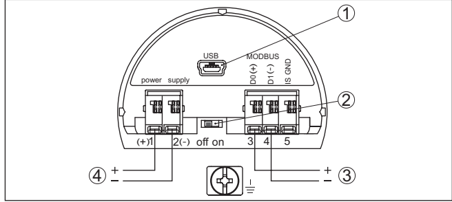
Res. 9: Bağlantı bölümü
