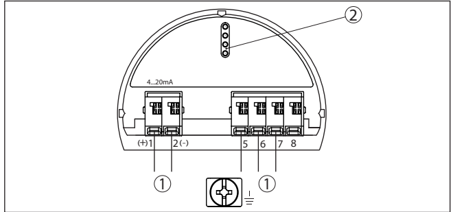
Res. 8: Elektronik bölgesi - iki hücreli gövde
