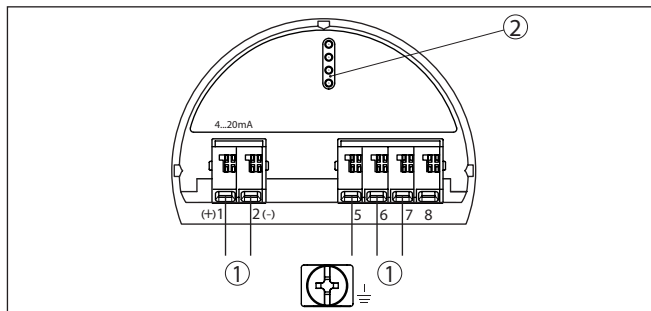
Fig. 8: Compartimento do sistema eletrônico - Caixa de duas câmaras
