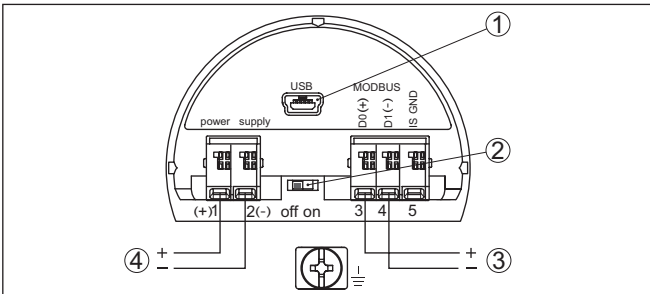
Fig. 9: Compartimento de conexões
