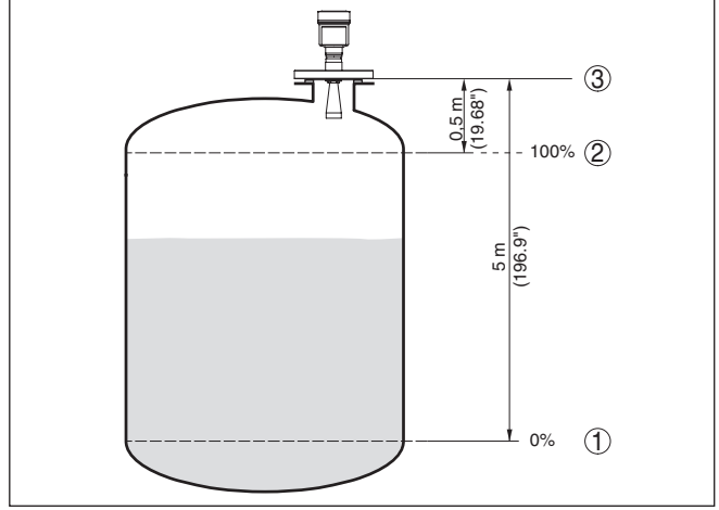
Res. 11: Min./Maks. seviye ayarı parametreleme örneği
