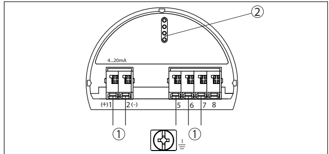
Res. 8: Elektronik bölümü - iki hücreli gövde
