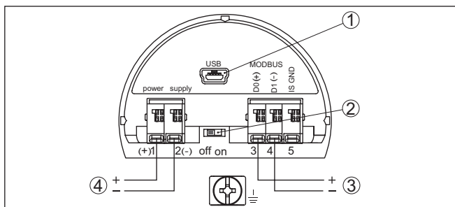
Rys. 9: Komora przyłączy
