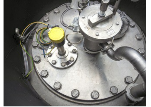
Radarlı seviye ölçüm cihazı VEGAPULS 64 tankın içindeki seviyeyi ölçüyor.
