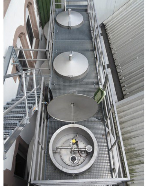
Depolama tanklarından birinin üzerinde bulunan radarlı seviye ölçüm cihazı VEGAPULS 64.
